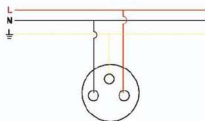
Схема цепи / Wiring Diagram
