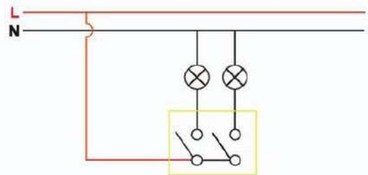
Схема цепи / Wiring Diagram
