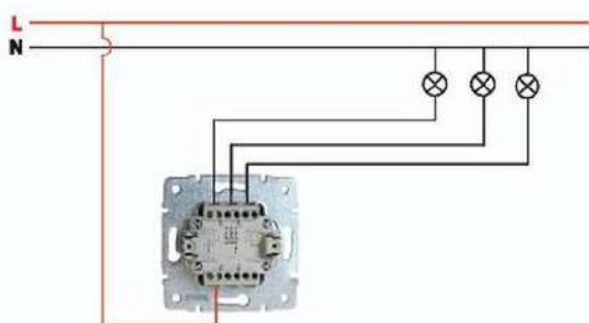
Схема подсоединения / Connection Diagram
