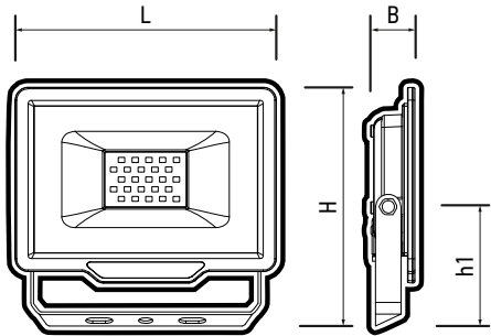
Рис. 1 Прожектор PFL-C3
