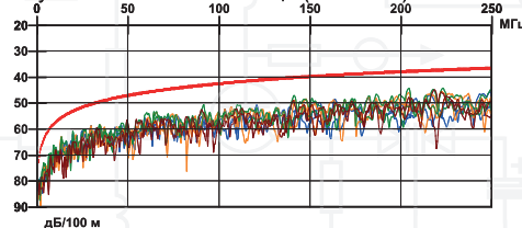
Возвратные потери (RL)
