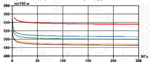
Время задержки сигнала (Delay)
