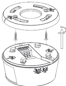
Рисунок 29 – Монтаж ДД 022 (LDD10-022-2000-K01)
