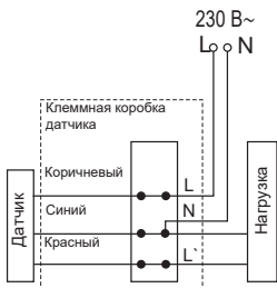
Рисунок 30 – Схема подключения датчиков типов ДД 013, ДД 015, ДД 016, ДД 040, ДД 042
