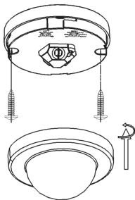
Рисунок 28 – Монтаж ДД 023 (LDD11-023-2000-001)
