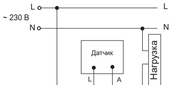
Рисунок 32 – Схема подключения датчика типа ДД 044
