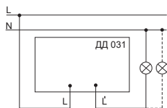
Рисунок 20 – Схема подключения датчика ДД 031
