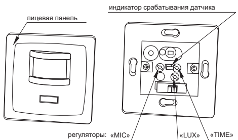
Рисунок 16 – Конструкция датчика движения ДД 035
