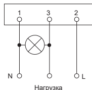
Рисунок 18 – Схема подключения датчика ДД 029
