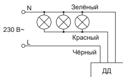
Рисунок 17 – Схема подключения датчика ДД 028
