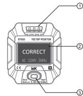
Тестер розеток ST03D
