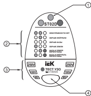
Тестер розеток ST02D
