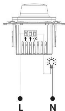
FI-D22-0250-X*; FI-D23-0550-X* (обычный)
