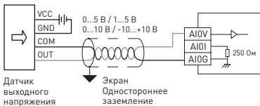
Рис. 5 – Подключение аналоговых входов (входной сигнал – напряжение)
