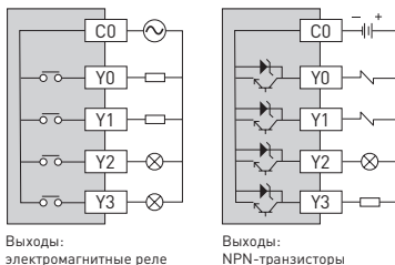
Рис. 4 – Подключение дискретных входов/выходов
