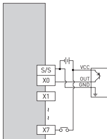
Выходы: PNP-транзисторы
