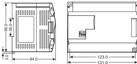
Рис. 3 – Габаритные размеры модулей REMF-D-20X20Y-R, REMF-D-20X20Y-N
