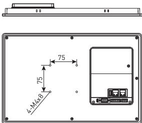
Рис. 4b – Размеры под крепление VESA для RSC-15E
