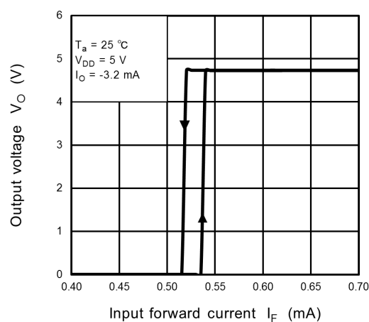
Fig. 13.2.10 V_O - I_F
