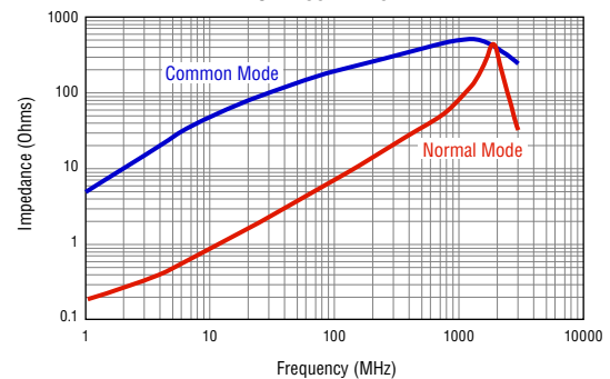
SRF4532TA-231Y
