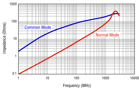
SRF4532TA-900Y
