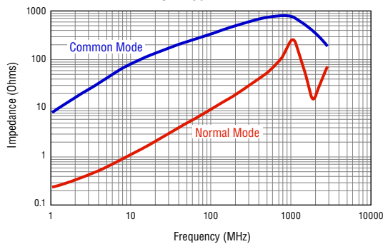
SRF4532TA-421Y
