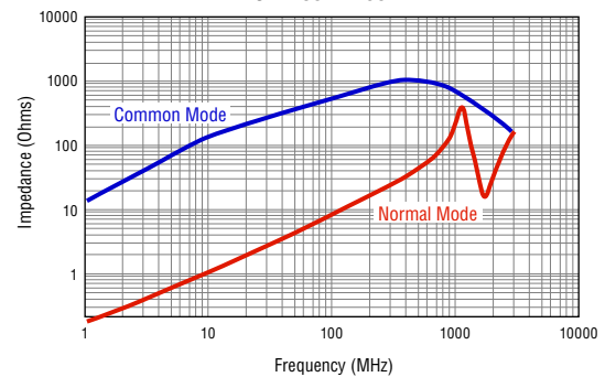
SRF4532TA-601Y
