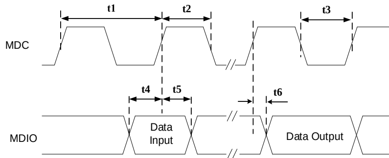
Figure 19. SMI (MDC/MDIO) Timing
