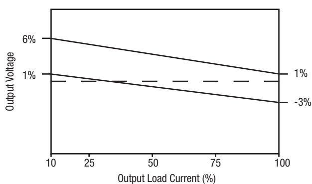
15V Output
