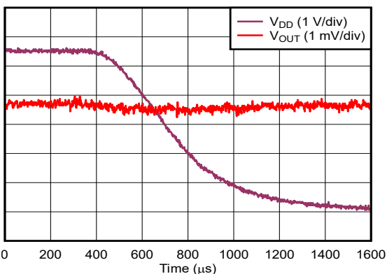
图 5-22. 输出电压建立时间：下降沿
