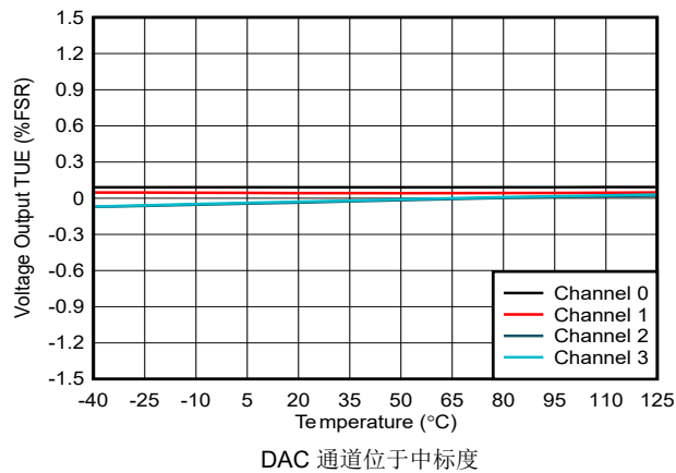
图 5-14. 电压输出 TUE 与温度间的关系
