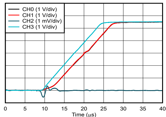
图 5-23. 电压输出上电干扰
