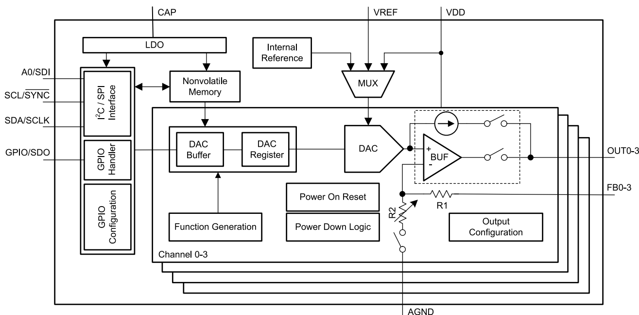
图 6-1. 功能方框图
