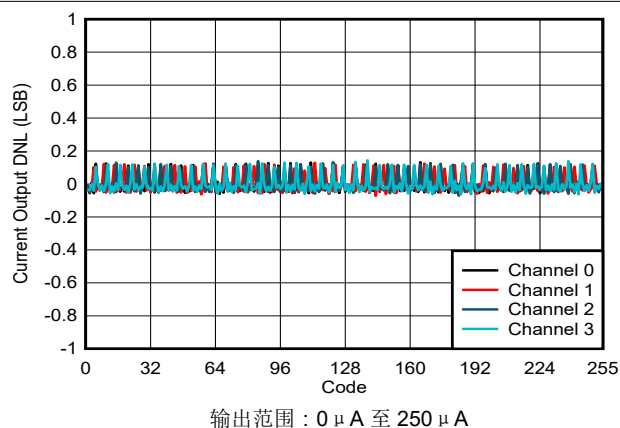
图 5-37. 电流输出 DNL 与数字输入代码间的关系
