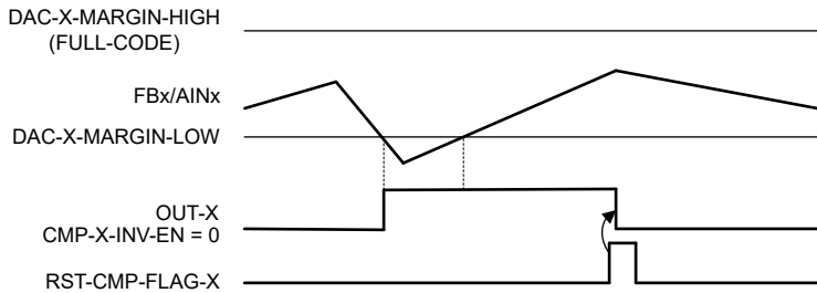
图 6-7. 具有高电平有效输出的锁存比较器
