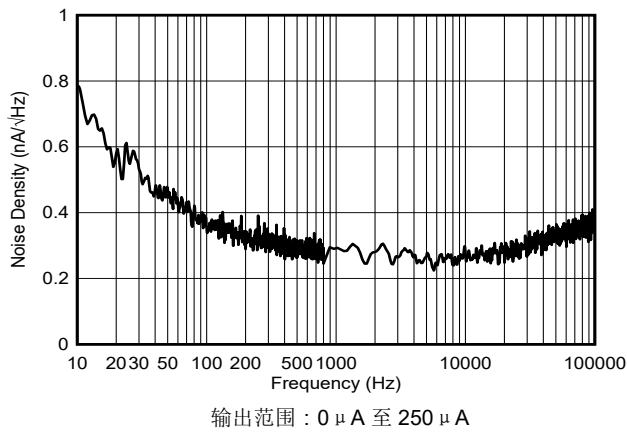
图 5-55. 电流输出噪声密度
