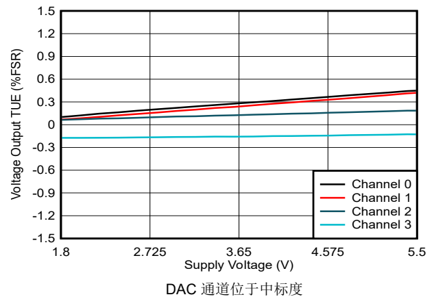
图 5-15. 电压输出 TUE 与电源电压间的关系
