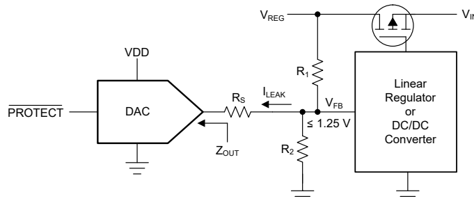
图 6-9. 高阻抗 (高阻态) 输出和 \overline{\text{PROTECT}} 输入
