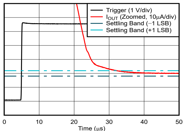
图 5-50. 输出电流稳定时间：下降沿（ \frac{3}{4} 至 \frac{1}{4} 标度）
