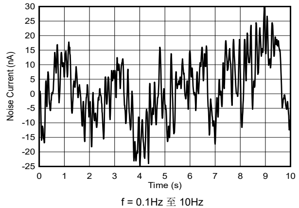
图 5-58. 电流输出闪烁噪声
