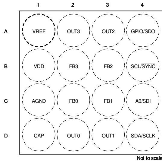
图 4-1. YBH 封装，16 引脚 DSBGA ( 顶视图 )
