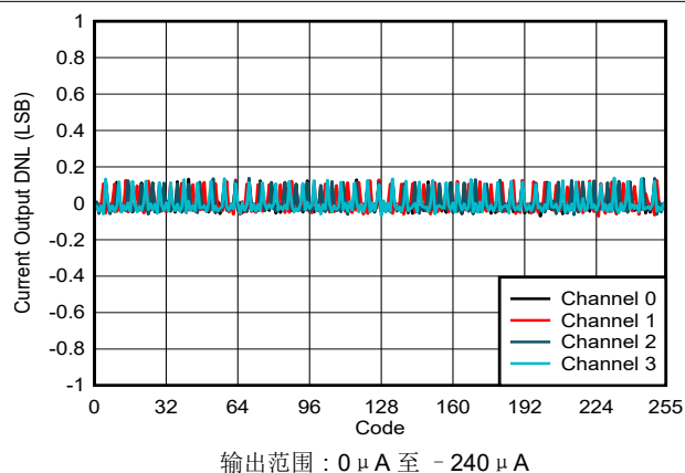
图 5-38. 电流输出 DNL 与数字输入代码间的关系
