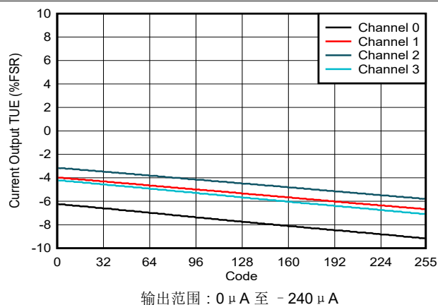
图 5-43. 电流输出 TUE 与数字输入代码间的关系
