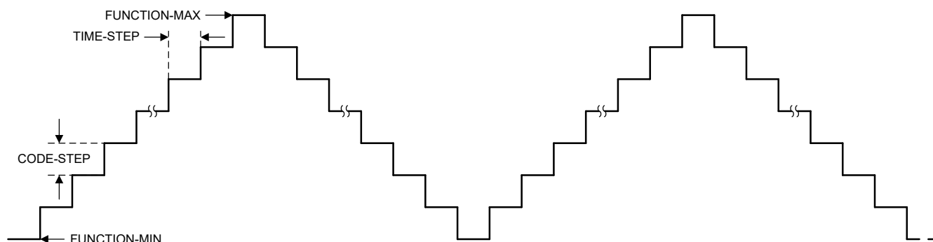
图 6-12. 三角波形
