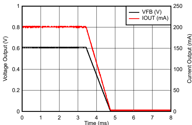
图 7-2. IOUT 和 VFB 导通至关断转换
