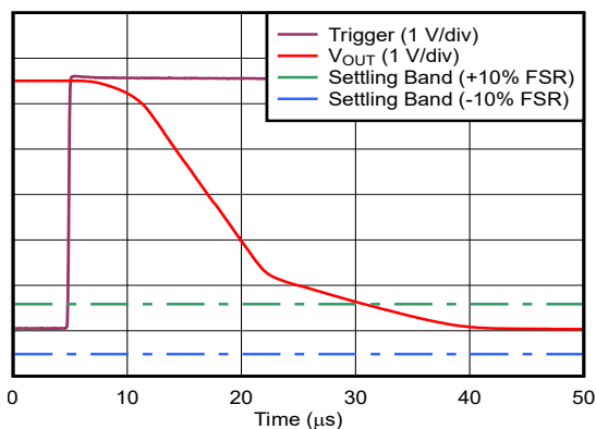
图 5-22. 输出电压建立时间：下降沿
