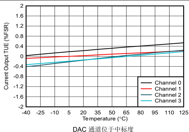
图 5-44. 电流输出 TUE 与温度间的关系
