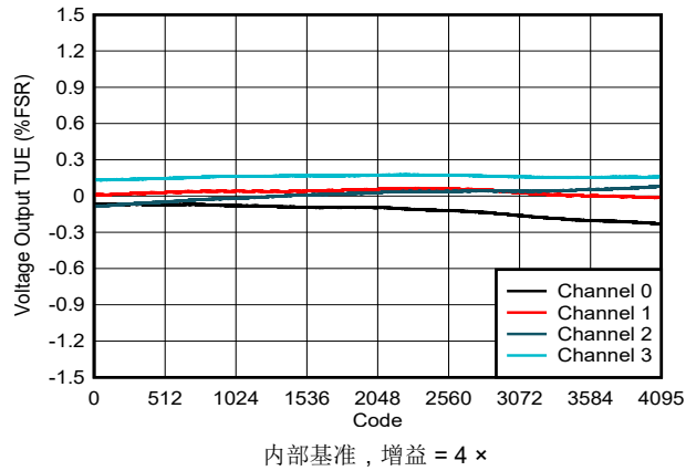
图 5-12. 电压输出 TUE 与数字输入代码间的关系
