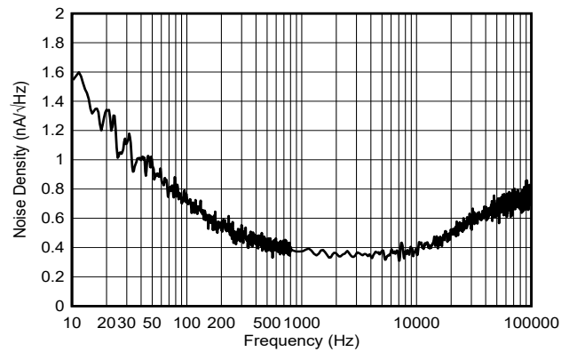
图 5-56. 电流输出噪声密度
