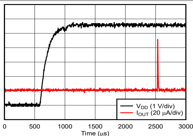
图 5-49. 输出电流稳定时间：上升沿（ \frac{1}{4} 至 \frac{3}{4} 标度）
