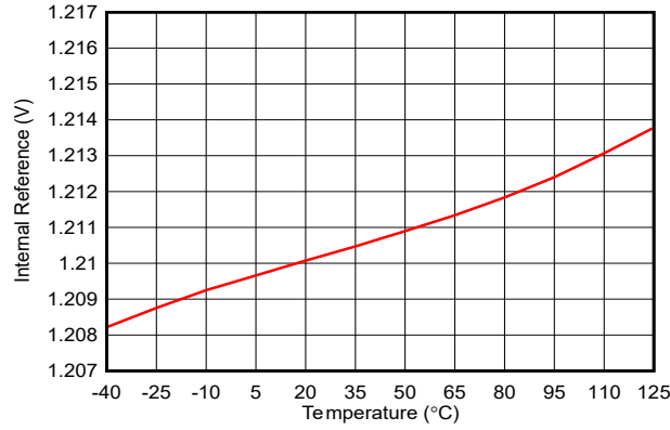
图 5-62. 内部基准与温度间的关系
