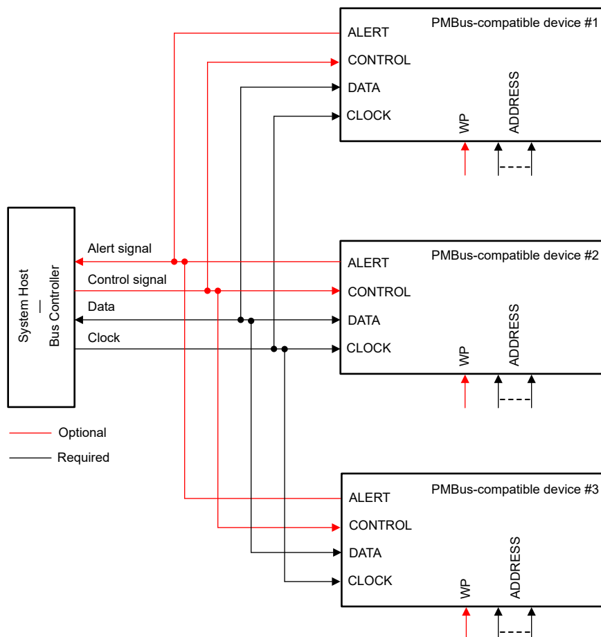
图 6-11. PMBus 连接
