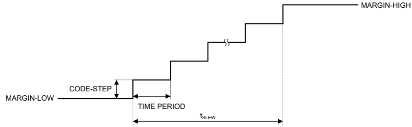
图 6-10. 可编程压摆率控制
