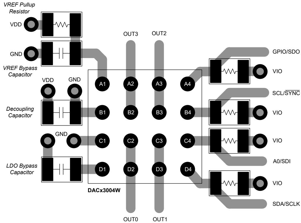
图 7-3. 布局示例
