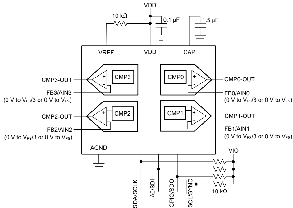
图 6-3. 比较器接口
