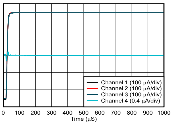
图 5-51. 电流输出上电干扰
