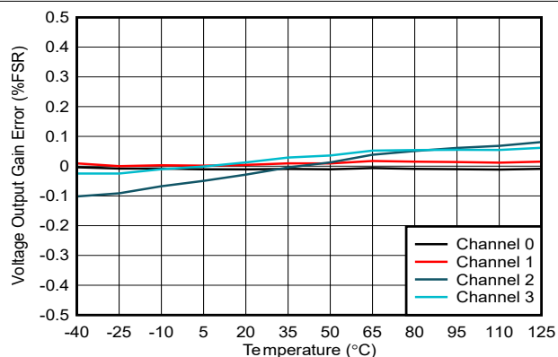
图 5-17. 电压输出增益误差与温度间的关系
