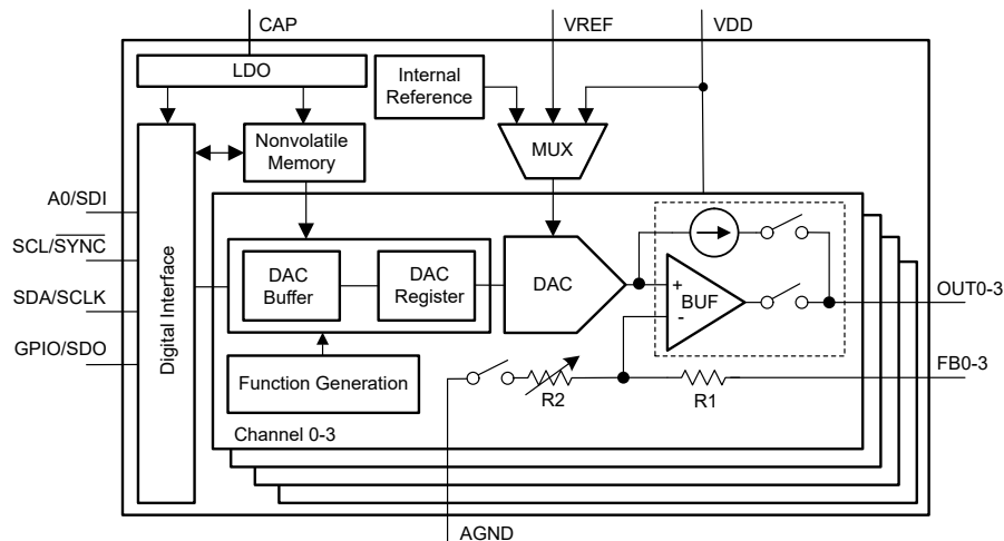
简化版方框图
