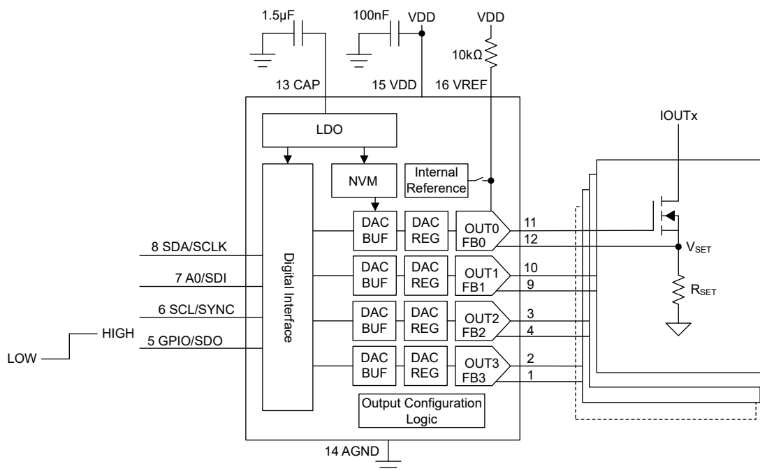
图 7-1. 电流源
