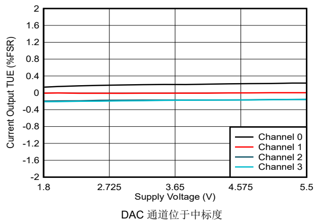
图 5-45. 电流输出 TUE 与电源电压间的关系
