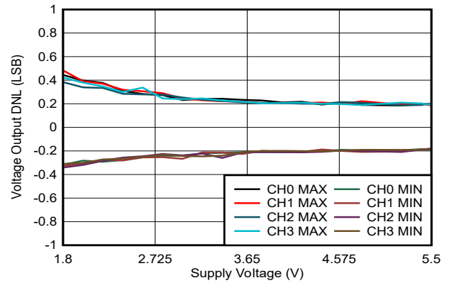
图 5-11. 电压输出 DNL 与电源电压间的关系
