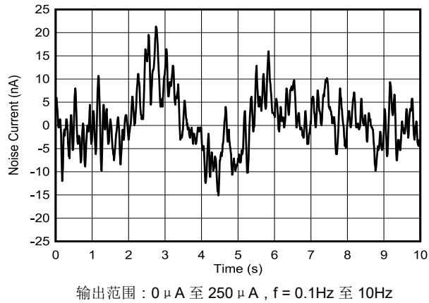
图 5-57. 电流输出闪烁噪声
