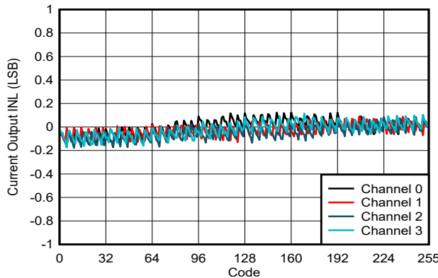
图 5-31. 电流输出 INL 与数字输入代码间的关系
