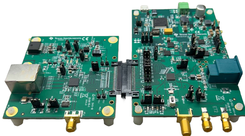
图 5-7. DP83TC818EVM-MC
