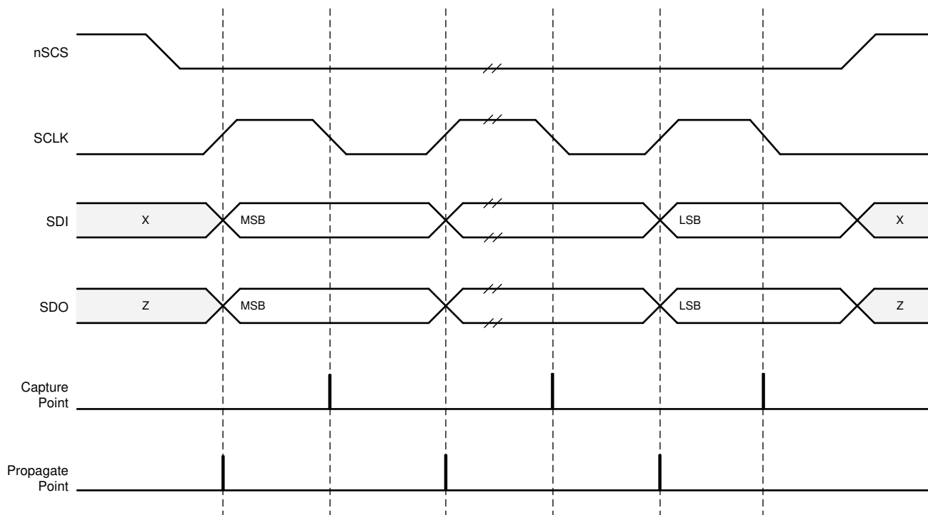
图 7-55. SPI 事务
