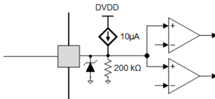
图 7-33. 三电平输入引脚图
