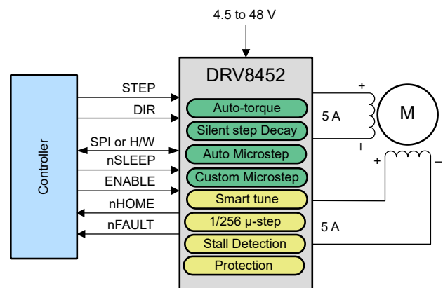
简化原理图
