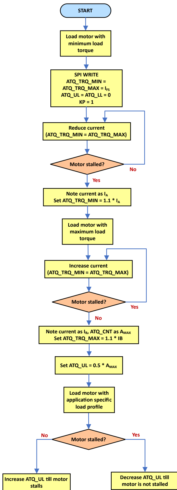
图 7-28. 选择 ATQ_TRQ_MIN、ATQ_TRQ_MAX、ATQ_UL、ATQ_LL
