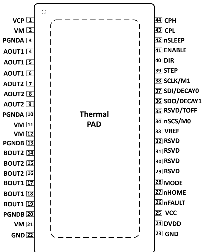
图 5-1. DDW 封装 ( 44 引脚 HTSSOP ) , 俯视图
