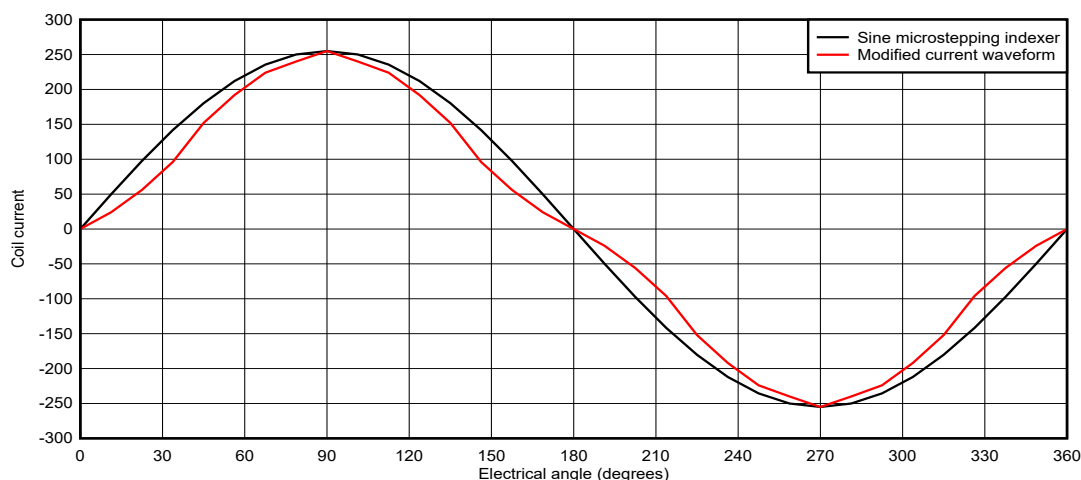
图 7-9. 可定制的微步进
