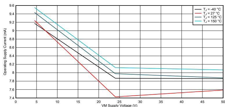
图 6-4. 工作电源电流, VCC = DVDD
