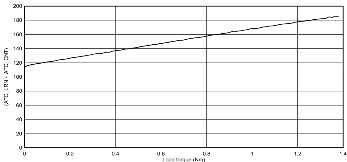
图 7-24. (ATQ_LRN + ATQ_CNT) 与负载转矩间的关系
