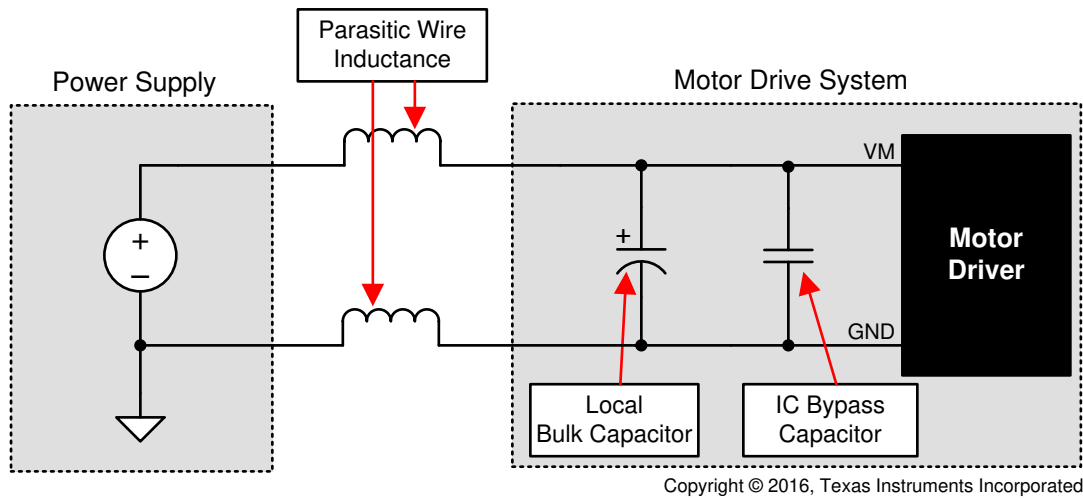
图 7-16. 带外部电源的系统设置示例
