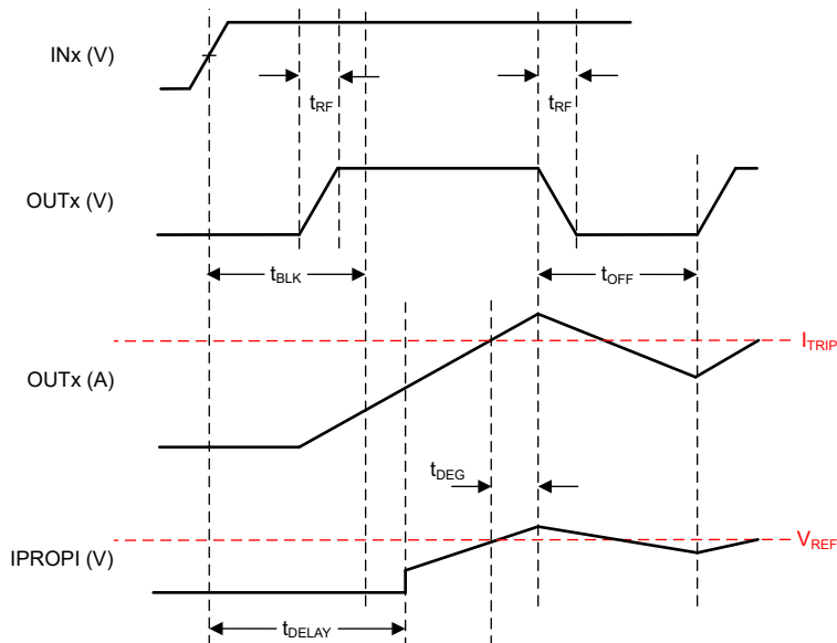
图 5-1. IPROPI 时序图
