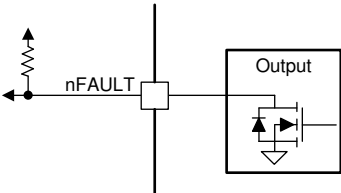
图 6-12. nFAULT 引脚
