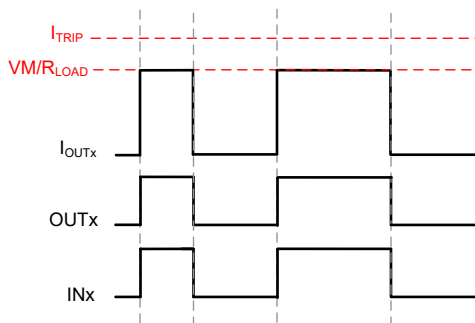
图 6-3. 电阻负载接地，逐周期控制
