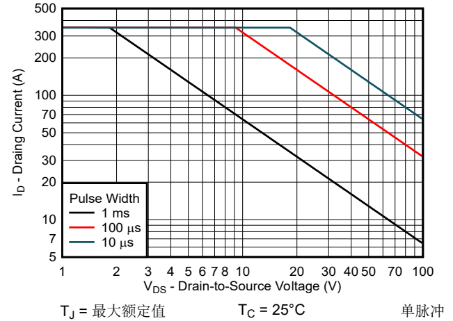
图 5-8. LMG3100R017 安全工作区
