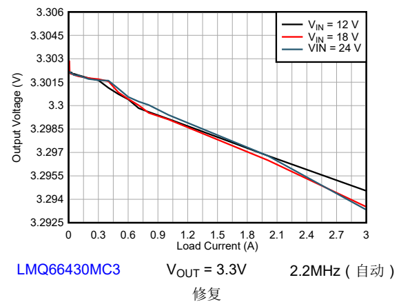
图 8-7. 线性 and 负载调整率
