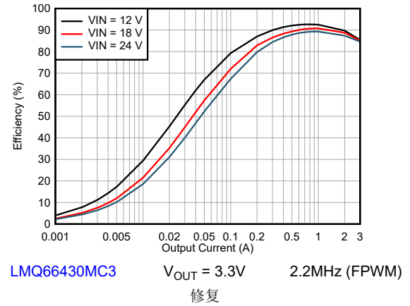
图 8-5. 效率
