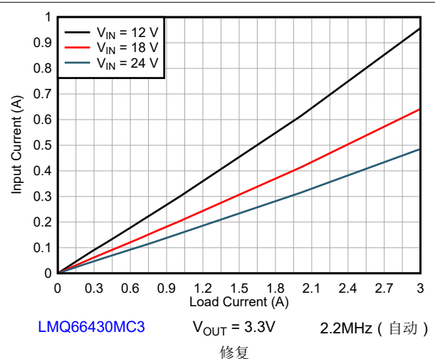
图 8-9. 输入电流与负载电流间的关系
