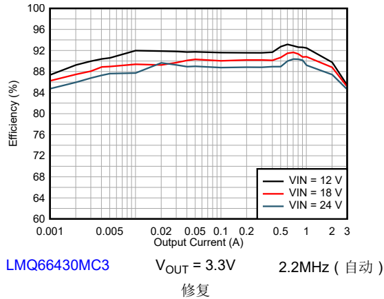
图 8-4. 效率
