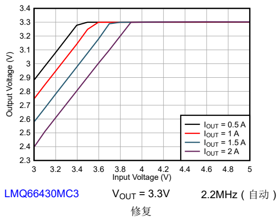
图 8-6. 压降
