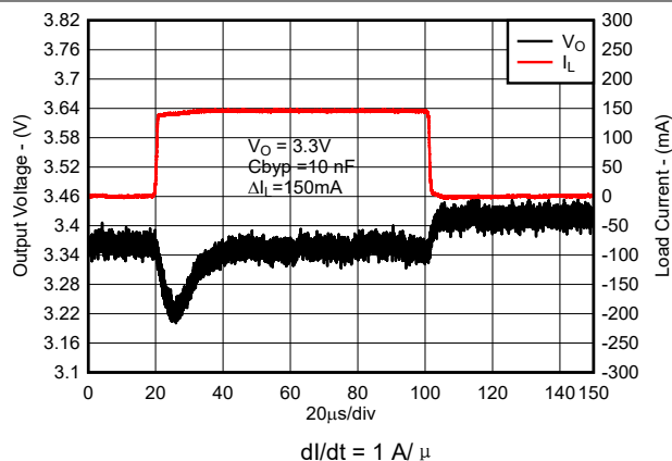
图 7-6. Load Transient for New Chip
