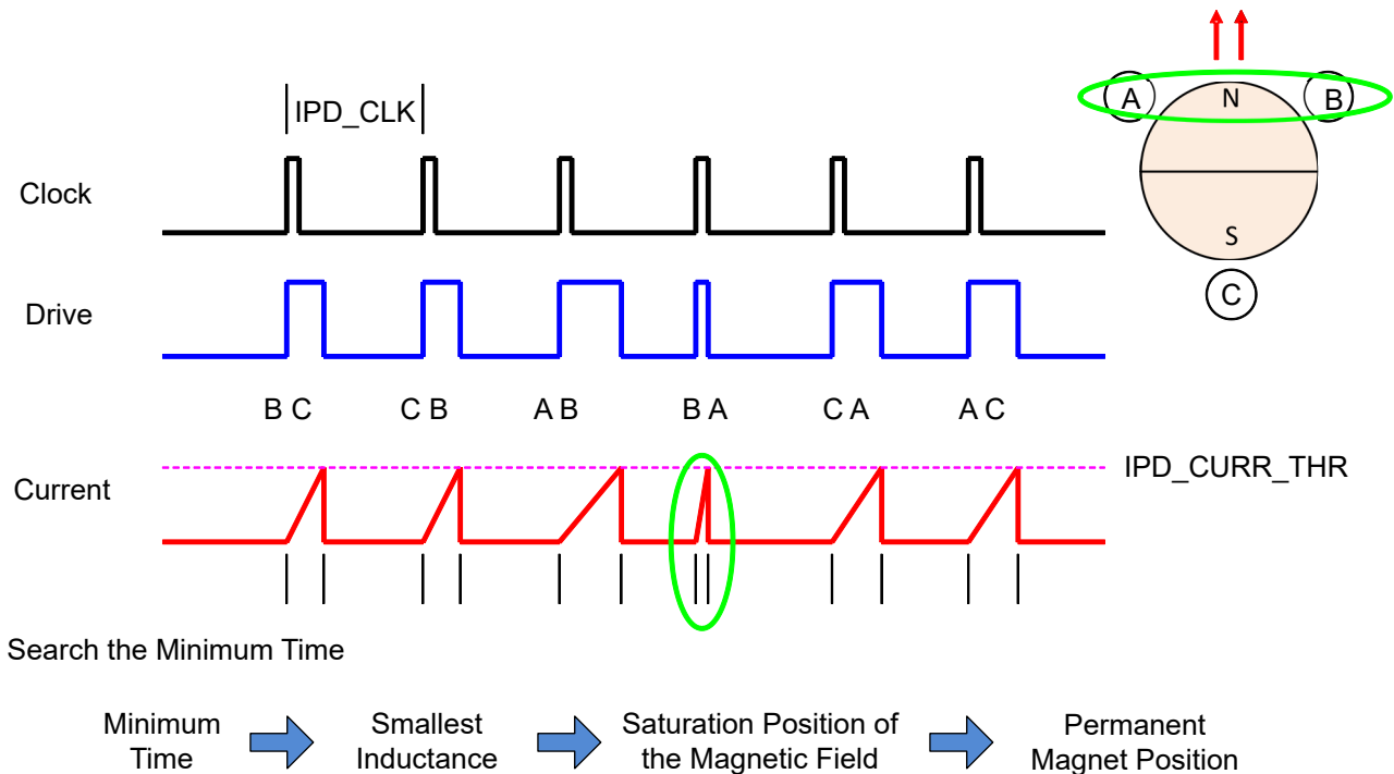
图 7-31. IPD 功能
