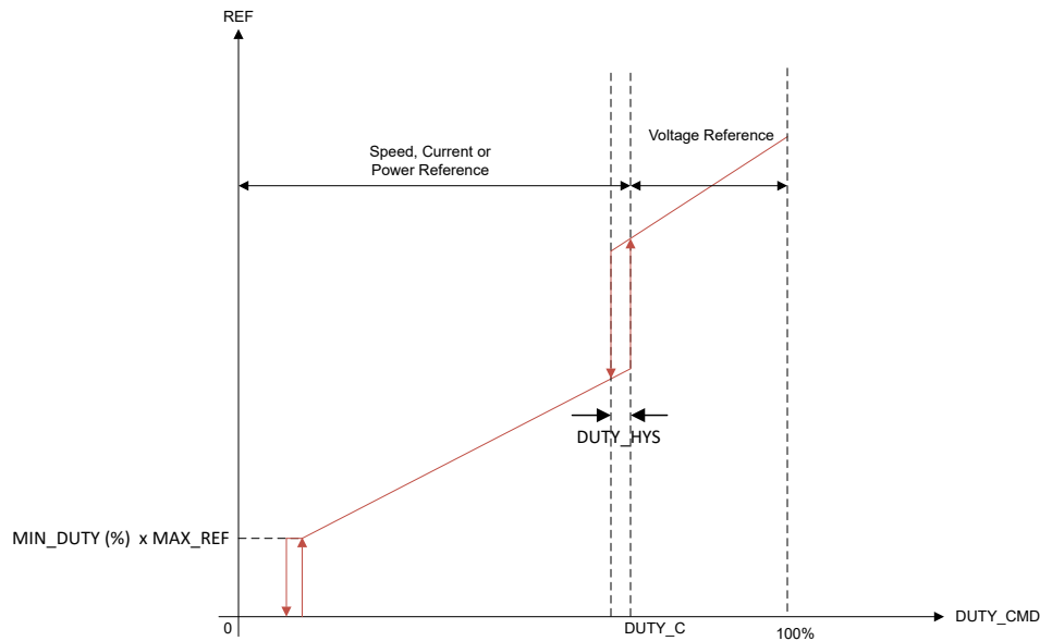
图 7-21. 多基准模式运行（当 VOLTAGE_MODE_CONFIG = 01b 时）
