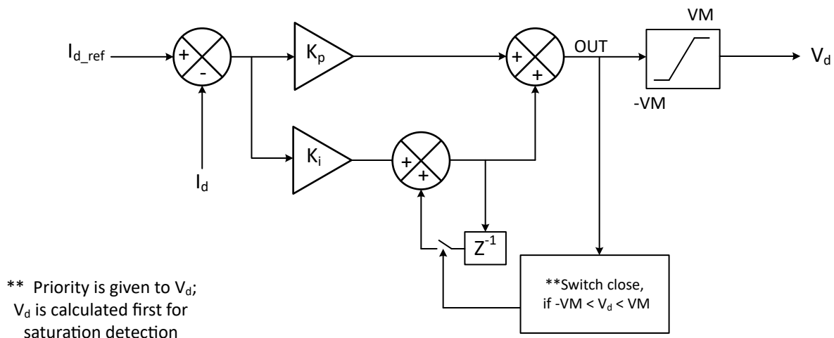
图 7-41. I_d 电流 PI 控制
