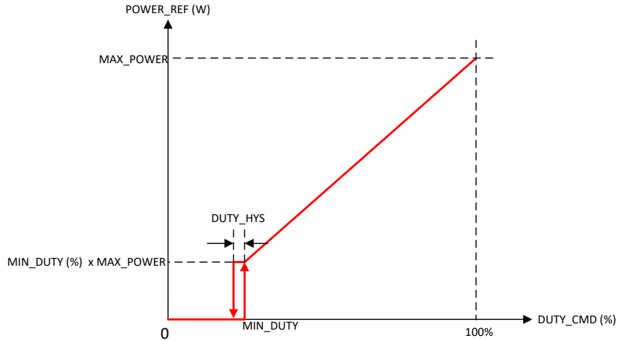
图 7-24. 功率基准传递函数
