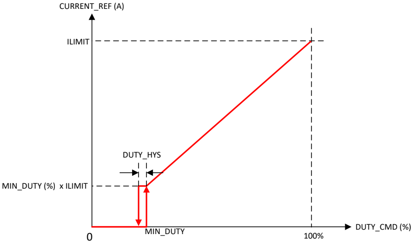
图 7-26. 电流基准传递函数
