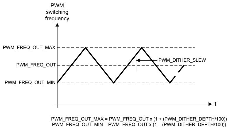
图 7-51. 三角 PWM 抖动
