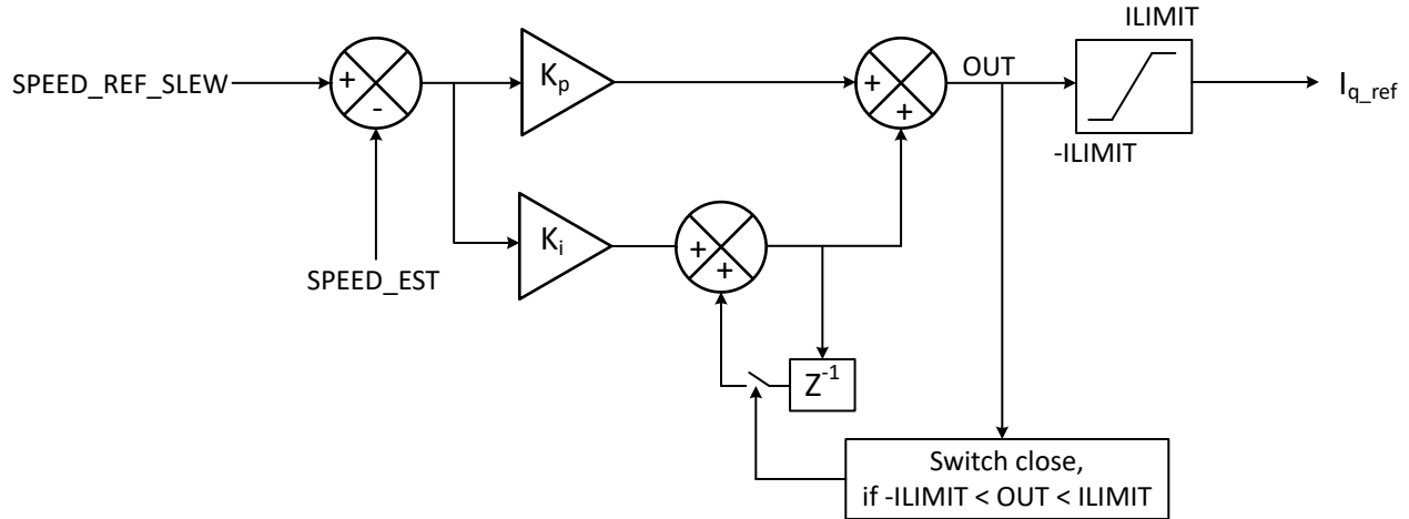
图 7-40. 速度 PI 控制
