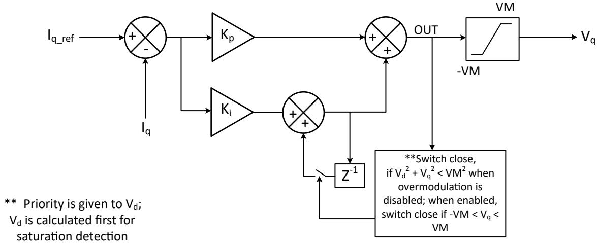
图 7-42. I_q 电流 PI 控制
