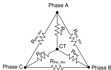
图 7-46. 电机电阻
