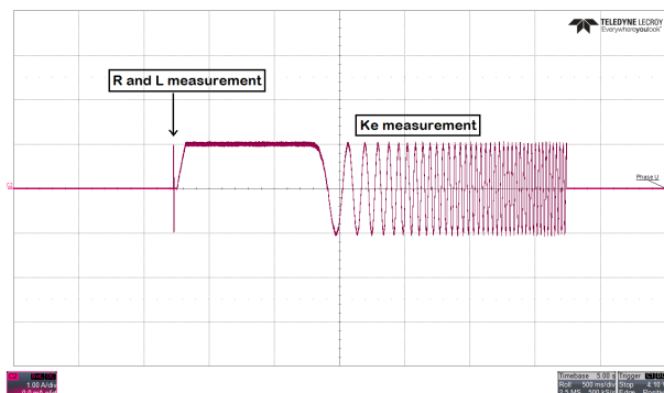
图 10-3. MPET - 相电流
