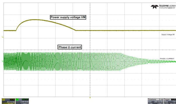
图 10-8. 禁用 AVS 时的电源电压和相电流波形
