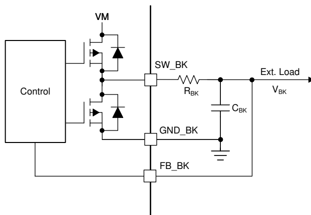
图 7-3. 降压 (电阻器模式)
