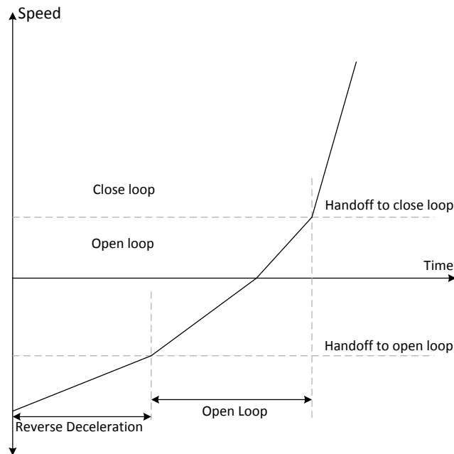
图 7-30. 反向驱动功能
