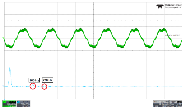
图 10-5. 相电流与 FFT - 死区时间补偿禁用时
