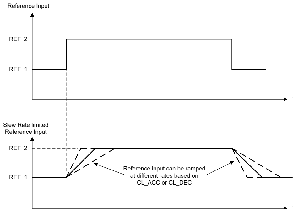
图 7-39. 闭环加速/减速压摆率
