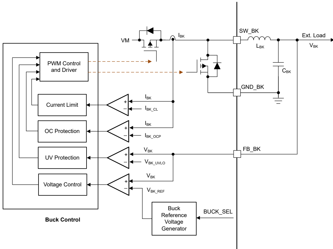
图 7-6. 降压运行和控制环路
