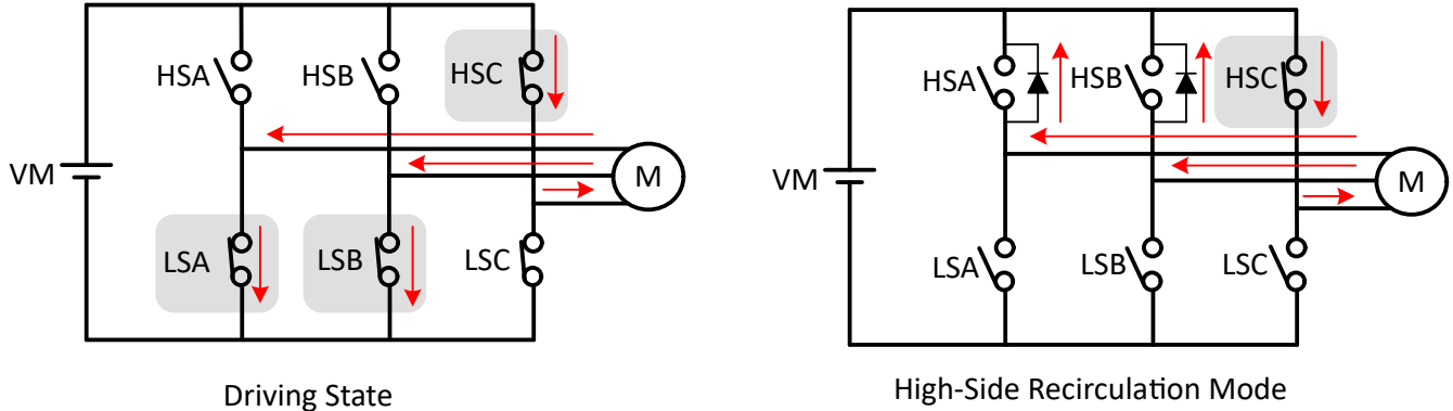
图 7-55. 高侧再循环
