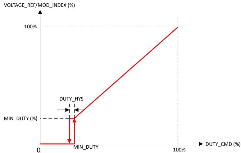
图 7-25. 电压基准传递函数
