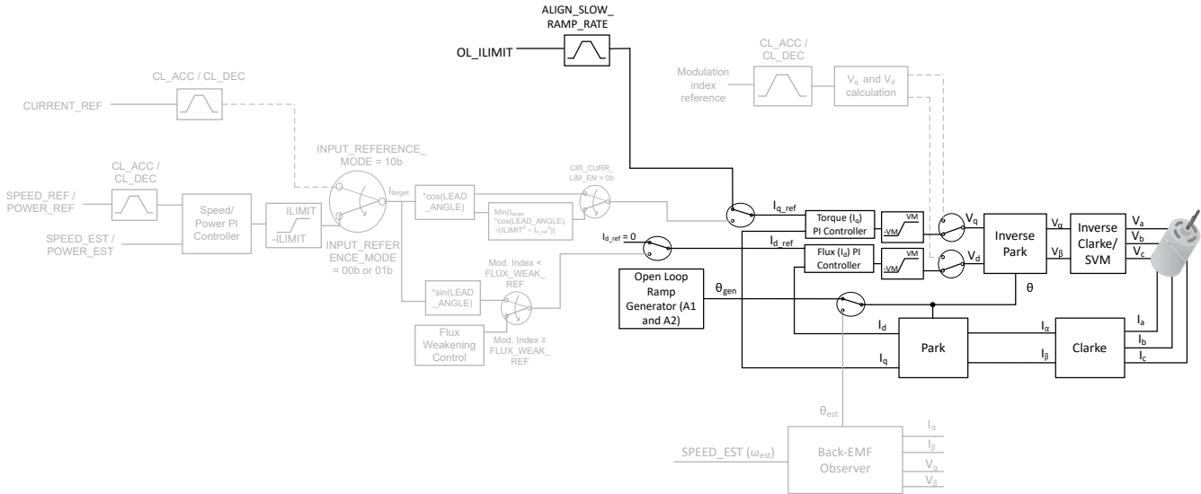
图 7-35. 开环
