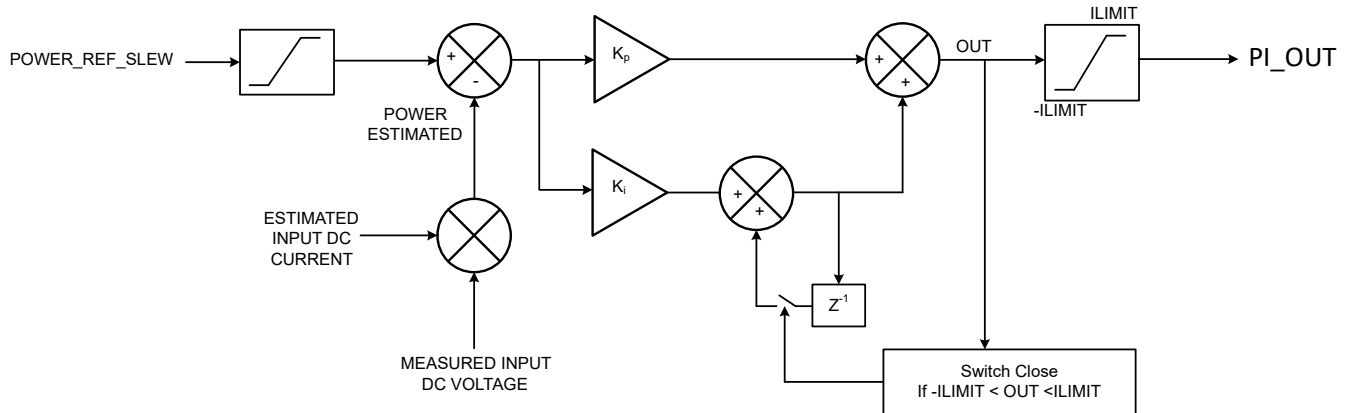
图 7-43. 闭环功率控制
