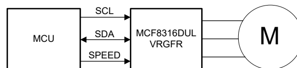
图 10-11. 采用 MCF8316DULVRGFR 的 IEC 60730 功能安全系统
