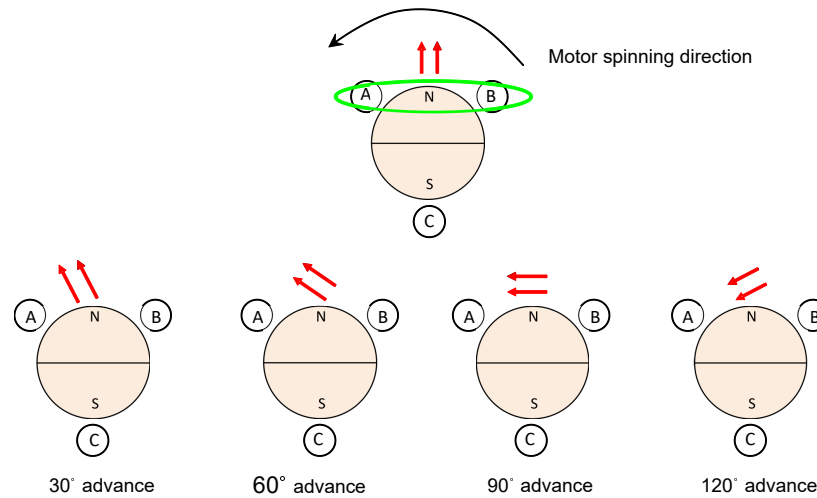
图 7-34. IPD 超前角度
