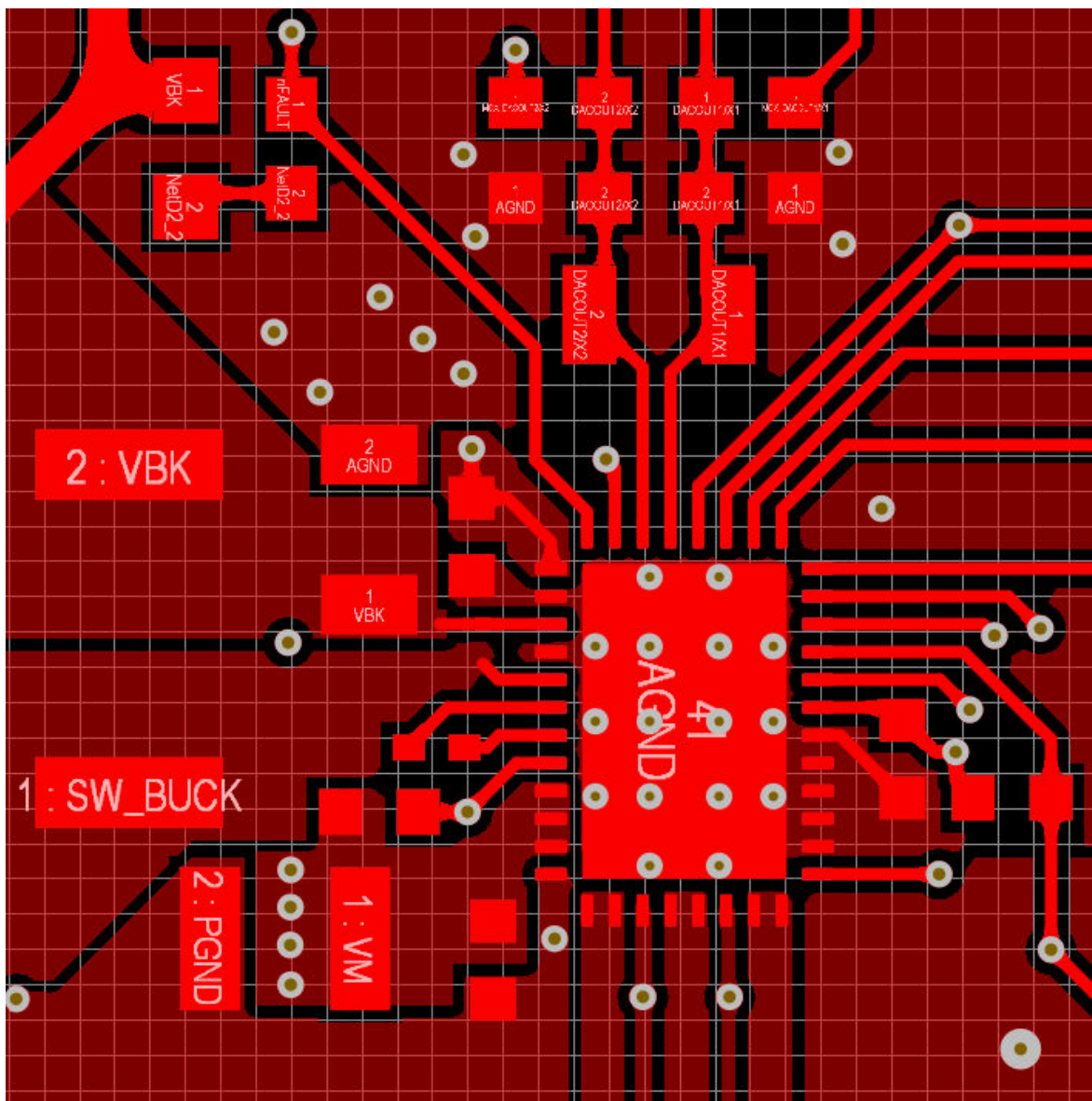
图 10-13. 推荐布局示例
