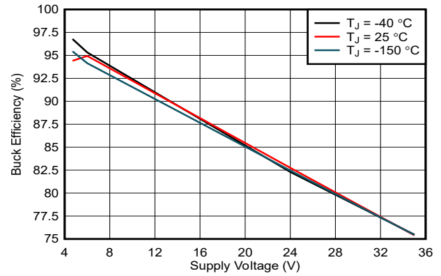
图 6-2. 降压稳压器在电源电压下的效率
