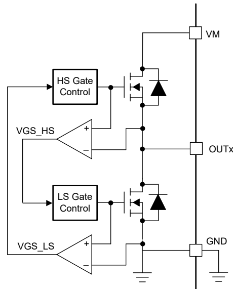
图 7-11. 跨导保护
