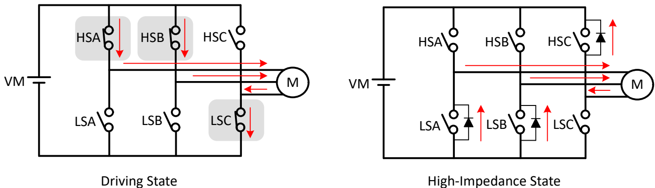
图 7-53. 滑行 ( 高阻态 ) 模式
