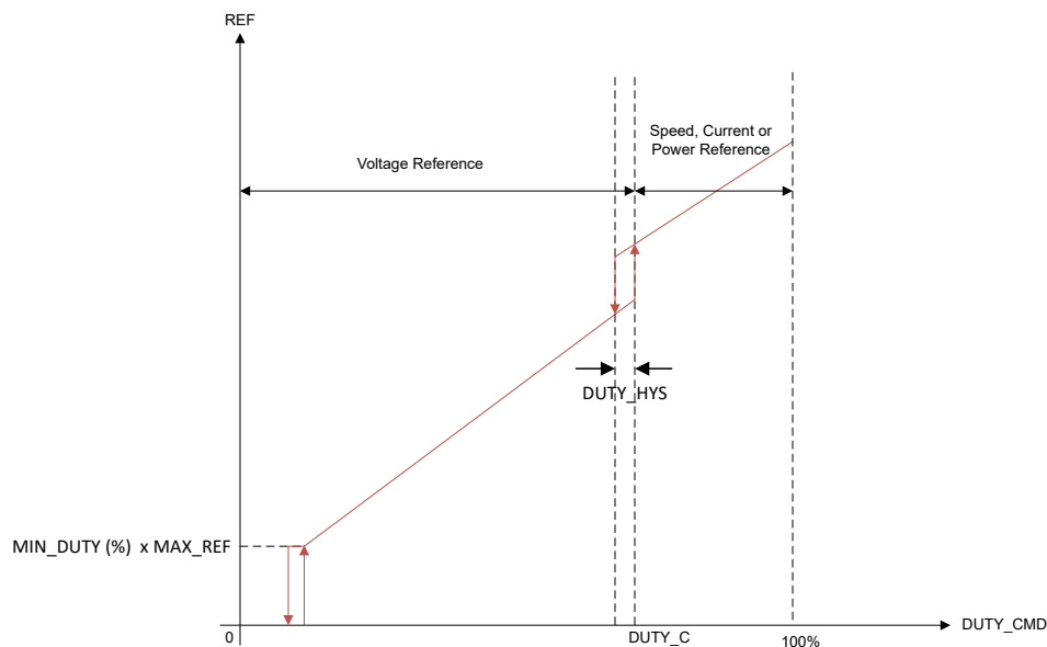
图 7-22. 多基准模式运行 ( 当 VOLTAGE_MODE_CONFIG = 10b 时 )
