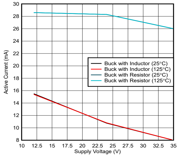
图 6-1. 电源电流与电源电压间的关系
