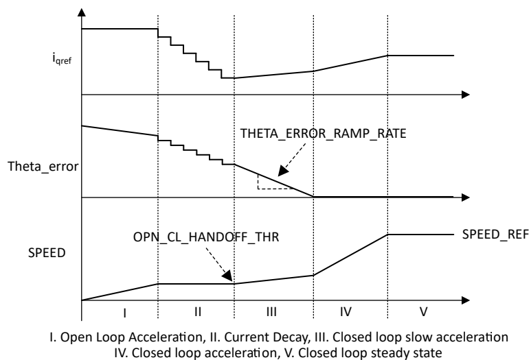
图 7-36. 开闭环转换中的控制序列
