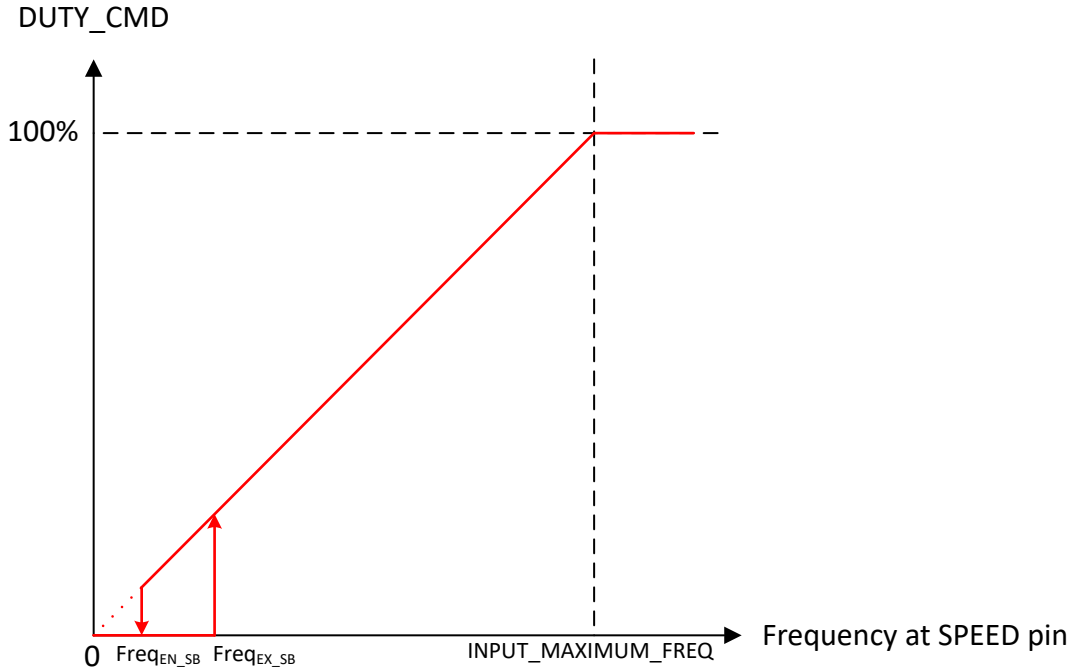
图 7-17. 频率模式速度控制
