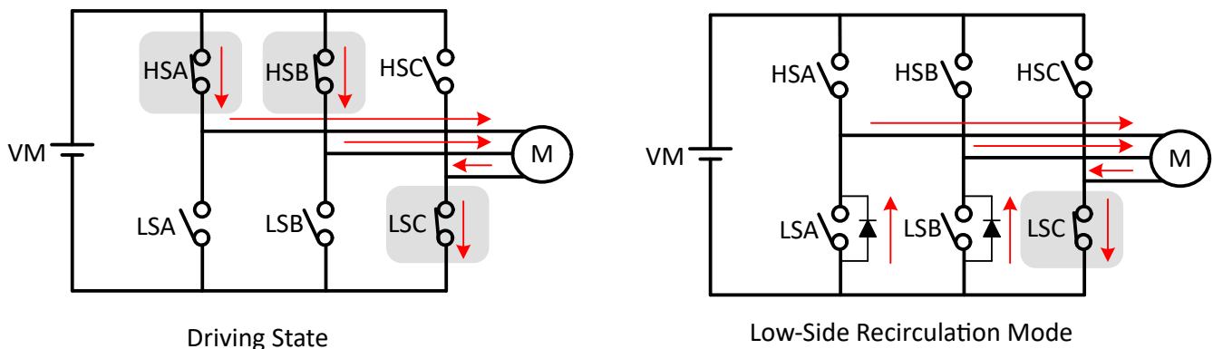
图 7-54. 低侧再循环
