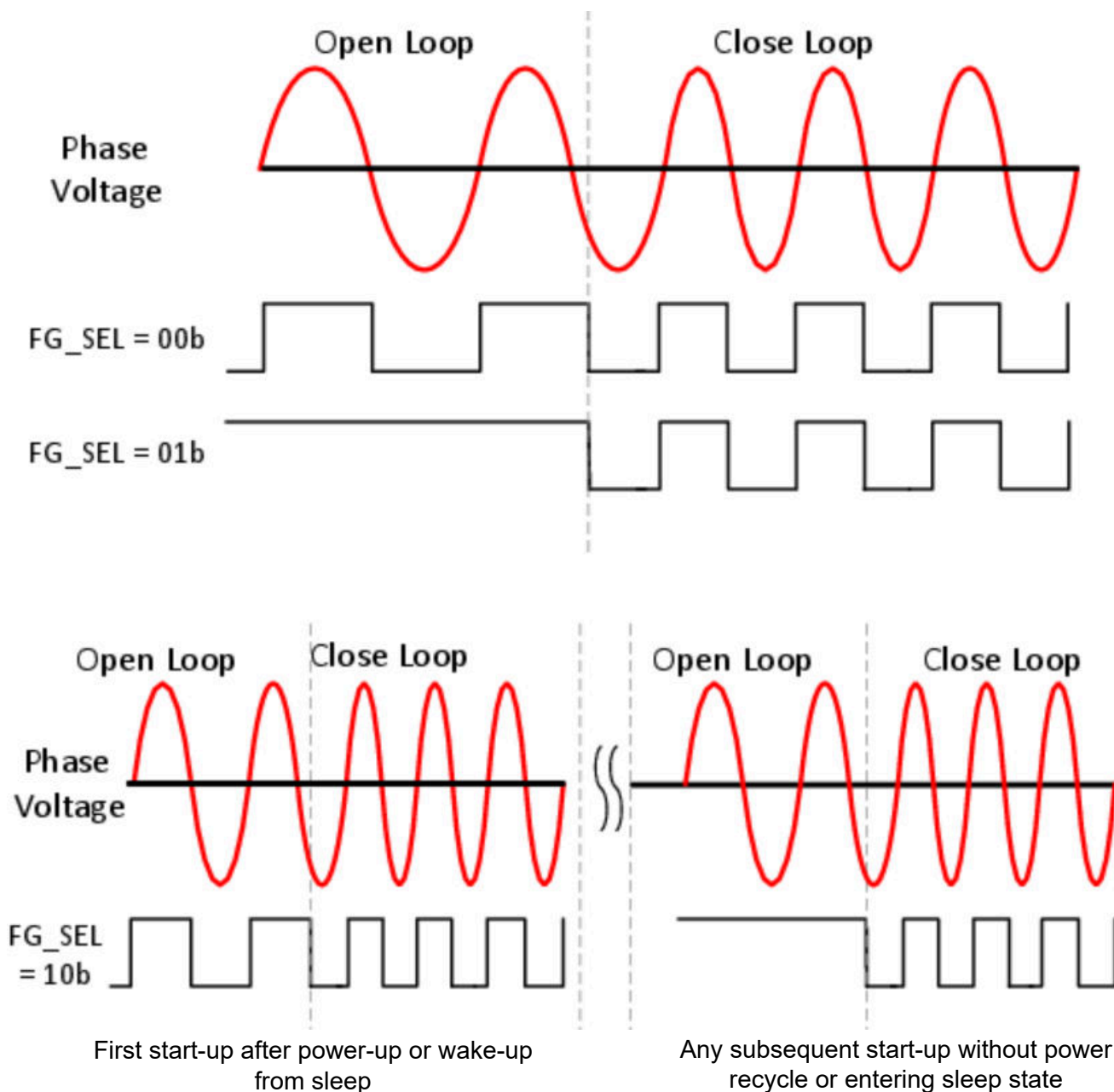
图 7-59. 开环期间的 FG 行为
