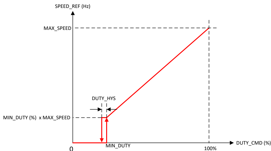
图 7-23. 速度基准传递函数
