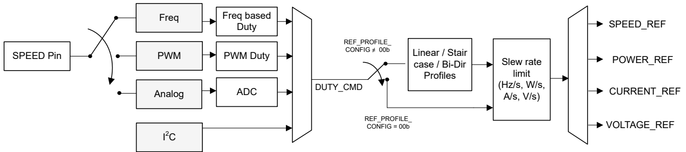
图 7-13. 多路复用基准输入命令
