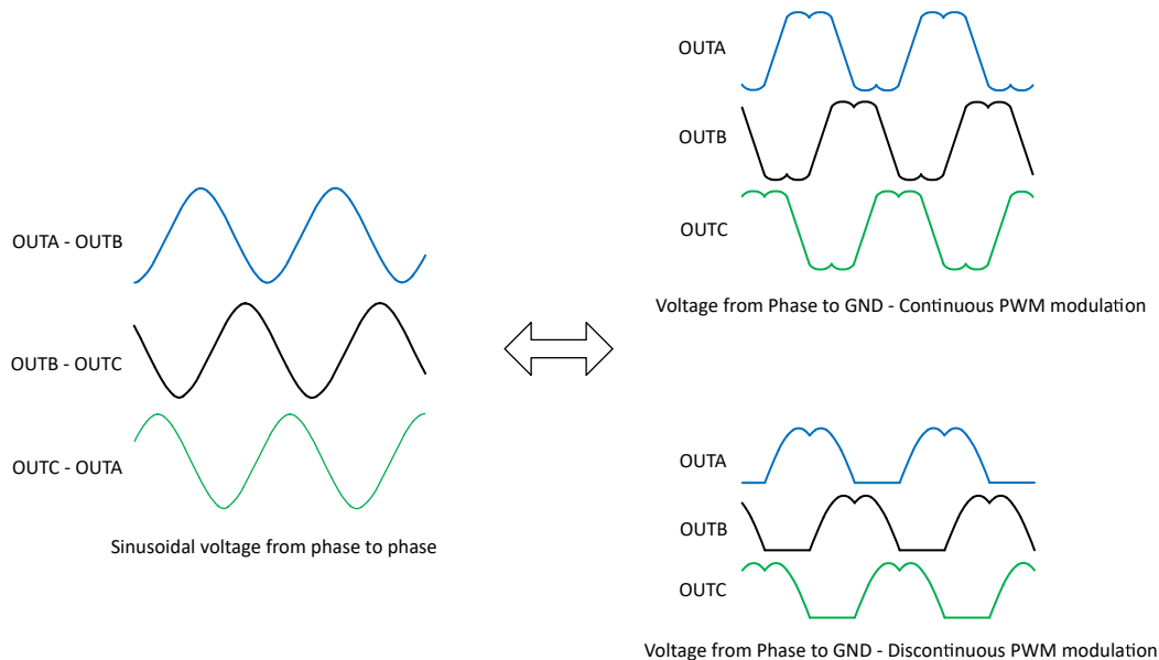
图 7-52. 连续和非连续 PWM 调制相位电压
