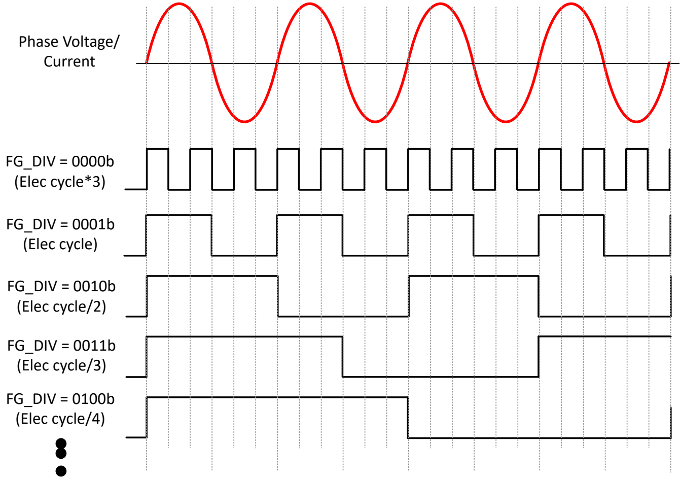
图 7-58. FG 分频器
