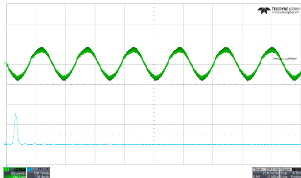
图 10-6. 相电流与 FFT - 死区时间补偿启用时
