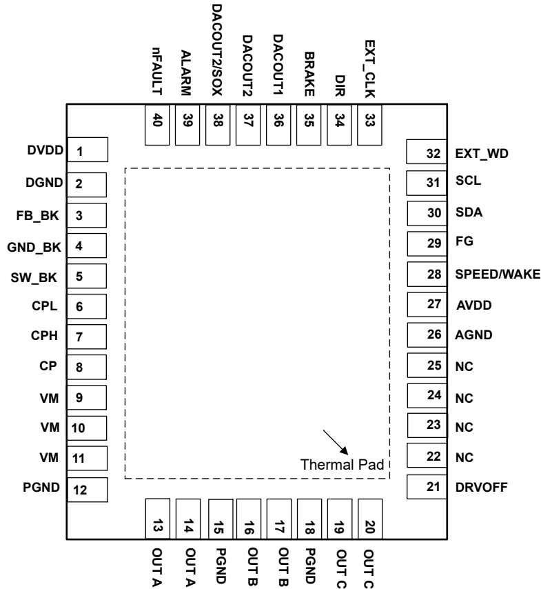
图 5-1. MCF8316D，40 引脚 VQFN（带有外露散热焊盘），顶视图
