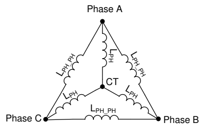
图 7-47. 电机电感
