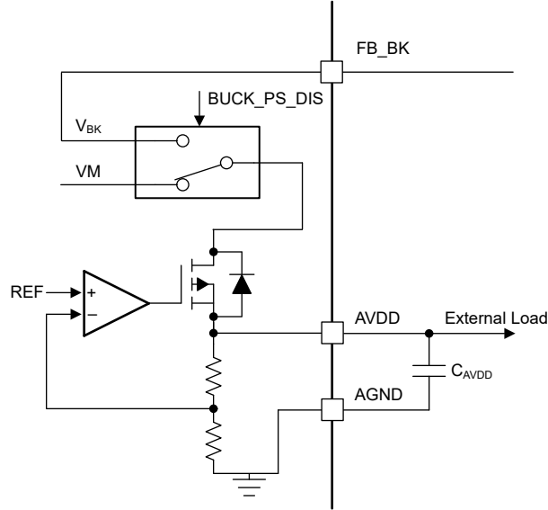
图 7-7. AVDD 线性稳压器方框图
