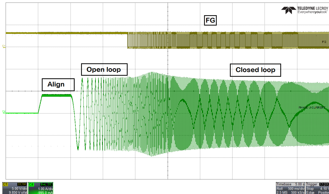
图 10-2. 电机启动 - FG 和相电流
