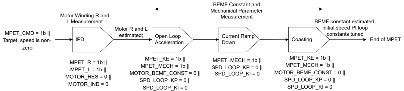
图 7-49. MPET 序列
