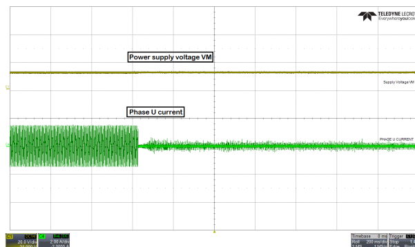
图 10-9. 启用 AVS 时的电源电压和相电流波形
