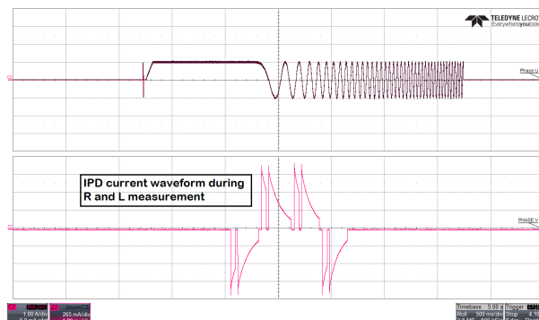
图 10-4. R 和 L 测量期间的 IPD 电流波形
