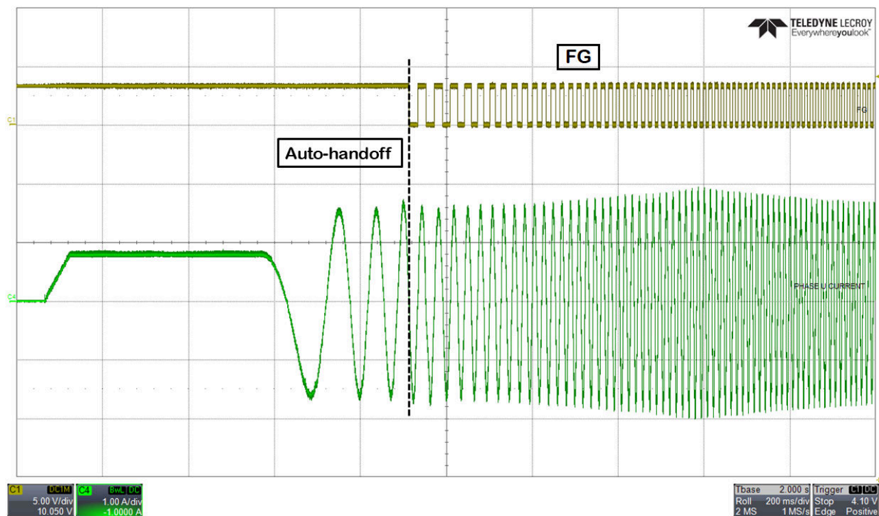
图 10-7. 自动转换
