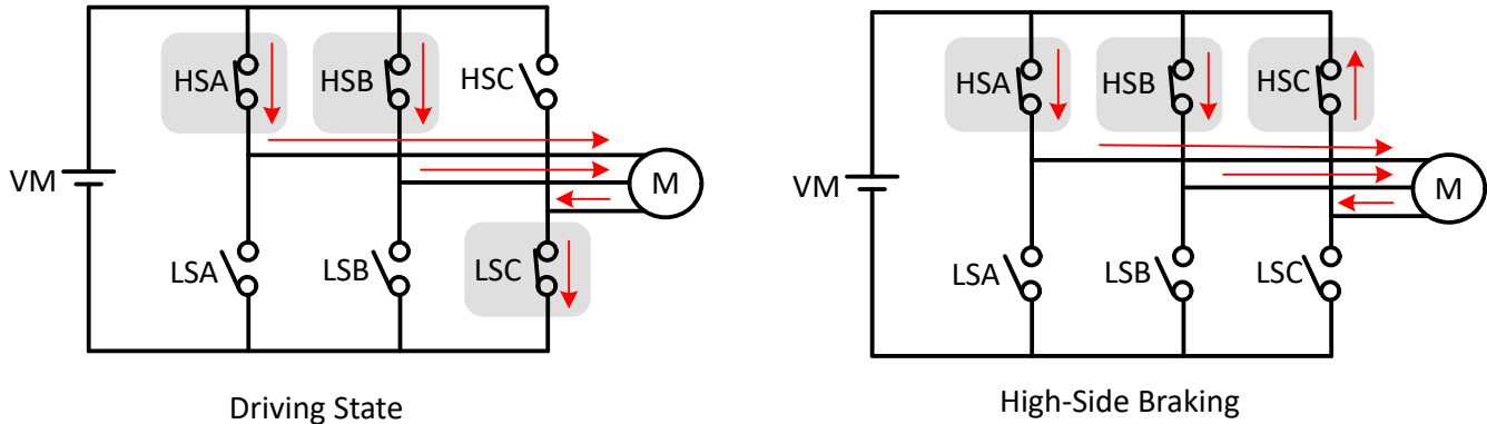
图 7-57. 高侧制动
