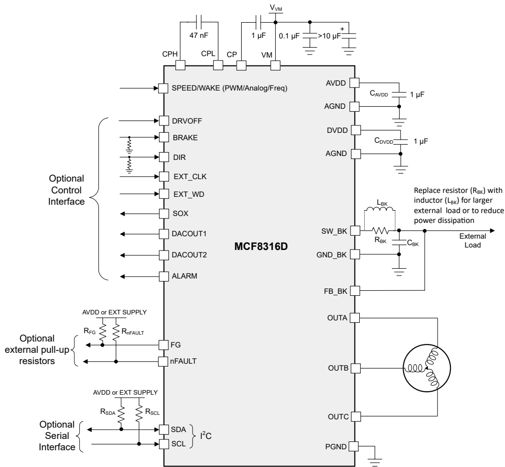
图 10-1. 示例应用原理图
