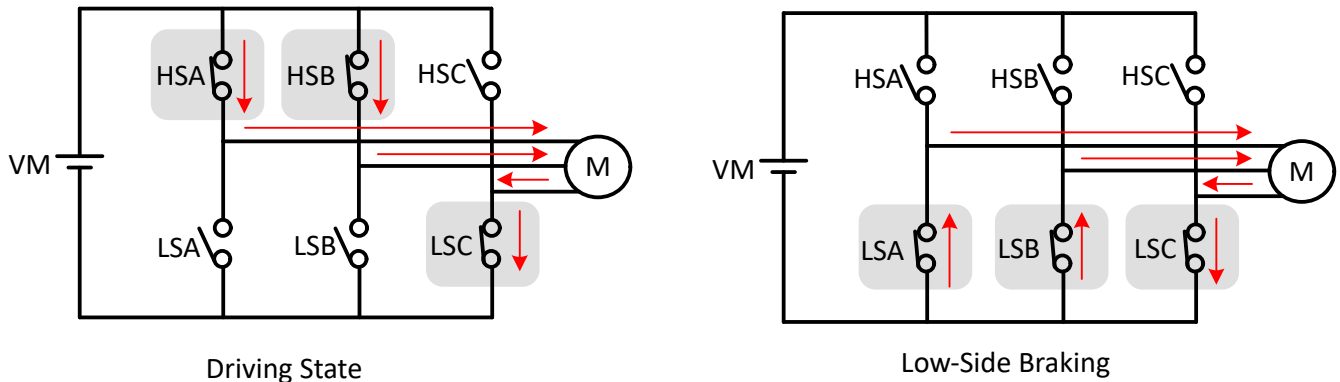
图 7-56. 低侧制动
