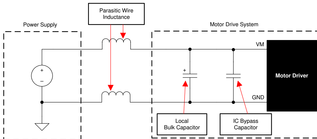
图 10-12. 带外部电源的电机驱动系统示例设置
