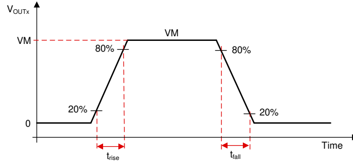
图 7-10. 压摆率时序
