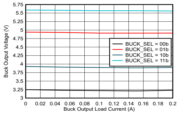
图 6-3. 降压稳压器输出电压随负载电流的变化
