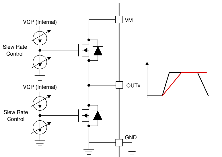
图 7-9. 压摆率电路实现
