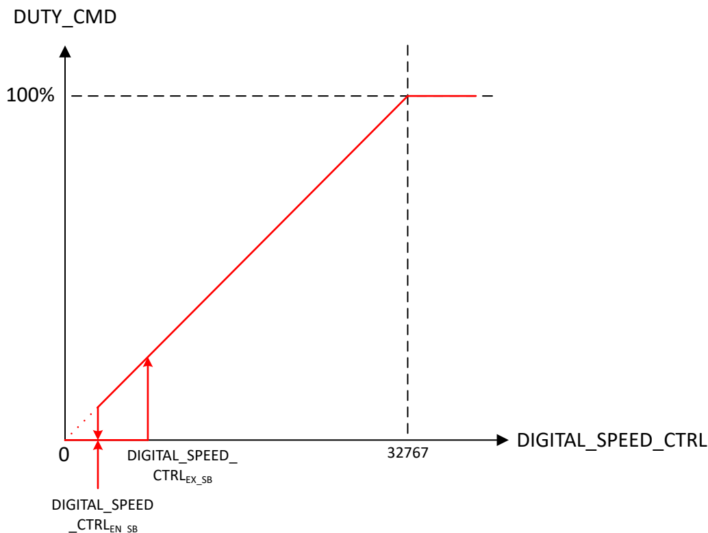
图 7-16. I2C 模式速度控制
