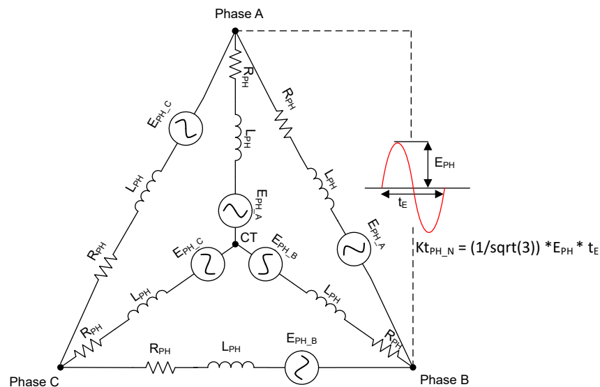
图 7-48. 电机反电动势常数
