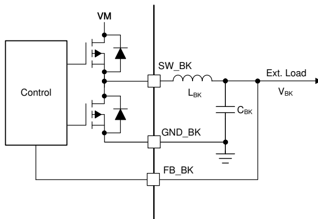
图 7-2. 降压 (电感器模式)
