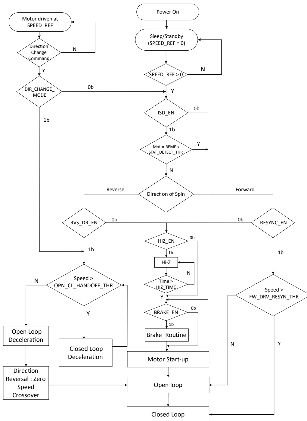
图 7-28. 电机启动序列
