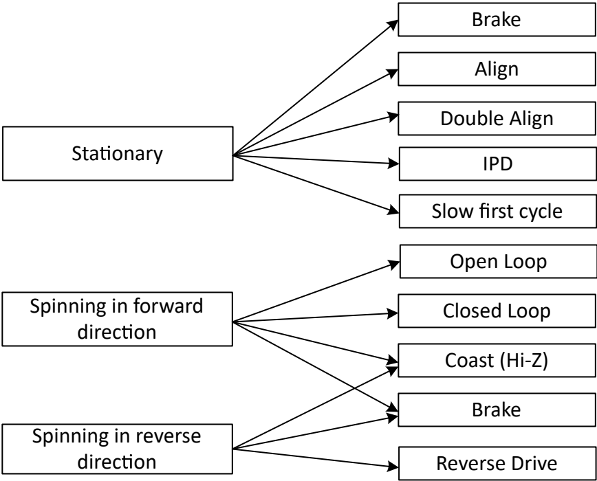
图 7-27. 在不同初始条件下启动电机
