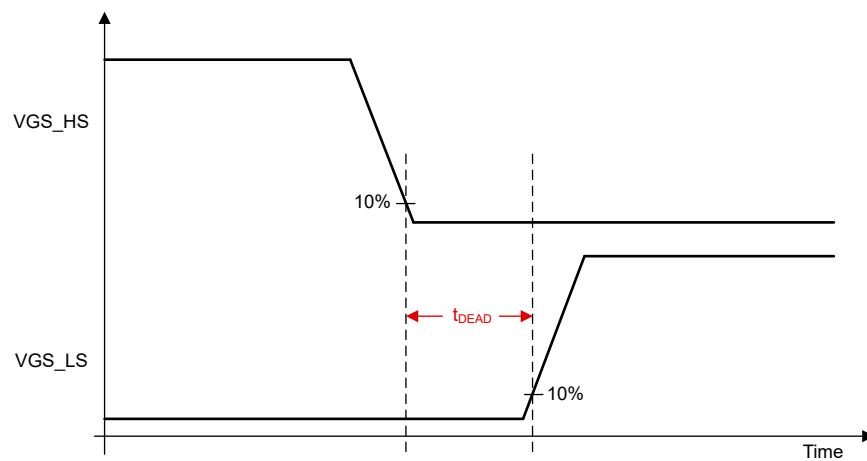
图 7-12. 死区时间
