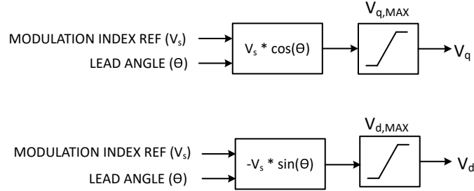
图 7-44. 开环电压控制
