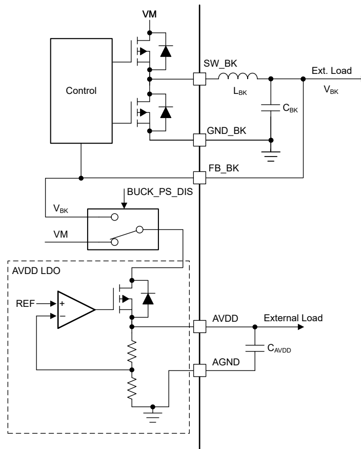
图 7-5. 混合模式降压稳压器中的 AVDD 电源时序
