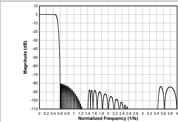
图 7-42. 线性相位内插滤波器幅度响应
