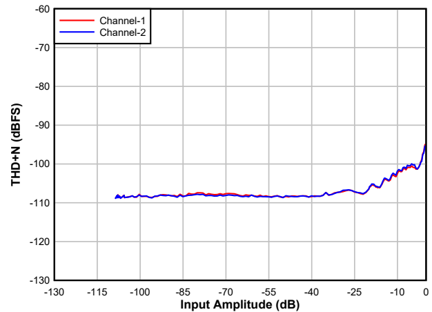
单端输出
