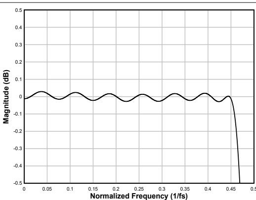
图 7-45. 线性相位内插滤波器通带纹波
