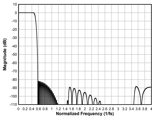
图 7-48. 线性相位内插滤波器幅度响应
