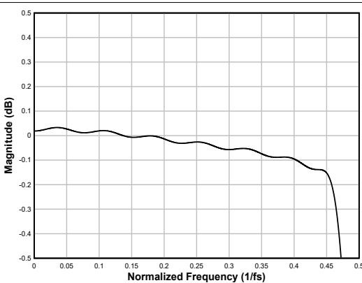
图 7-43. 线性相位内插滤波器通带纹波
