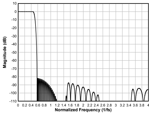
图 7-46. 线性相位内插滤波器幅度响应
