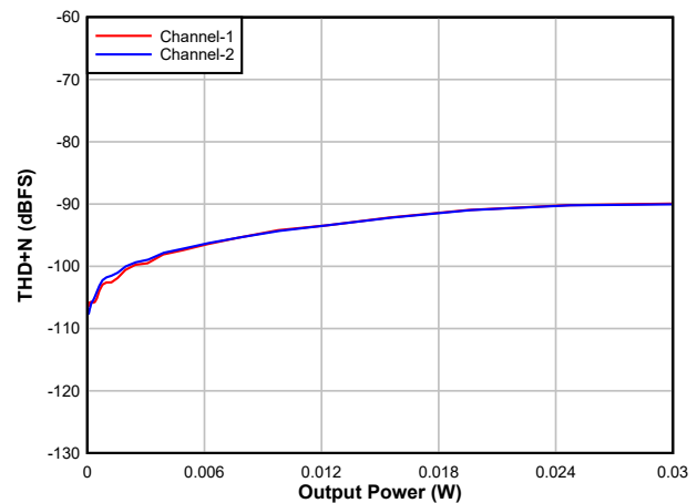
伪差分输出, 32 \Omega 耳机负载
