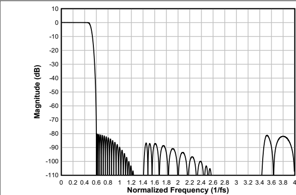
图 7-17. 线性相位抽取滤波器幅度响应
