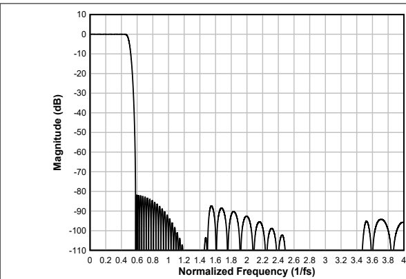
图 7-44. 线性相位内插滤波器幅度响应
