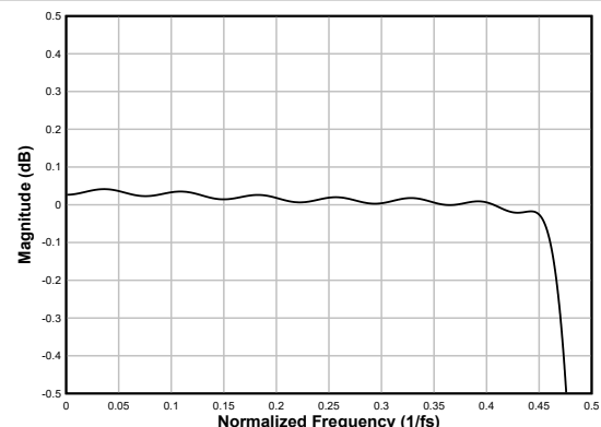
图 7-16. 线性相位抽取滤波器通带纹波
