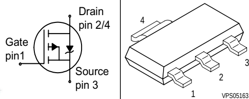
PG-SOT223
