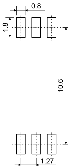
図 15.1 リードフォーミング, テーピングオプション (LF4), (TP4)
