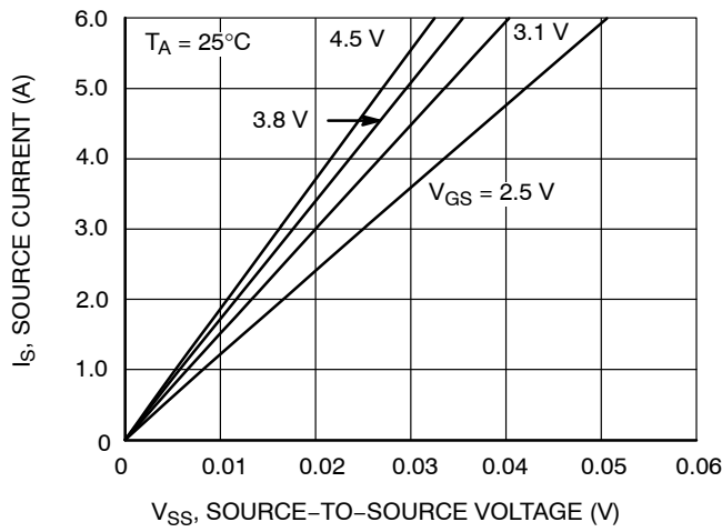
Figure 8. I_S - V_{SS}
