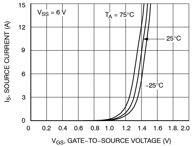
Figure 9. I_S - V_{GS}
