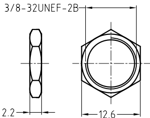
METAL NUT
