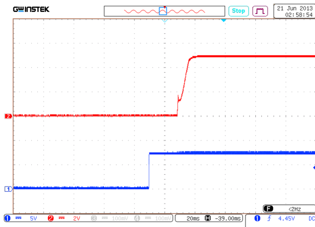
Рис. 31. Установление U_{ВЫХ.НОМ} с момента подачи сигнала ДУ (соединение выводов «ДУ» и «-ВХ»).
