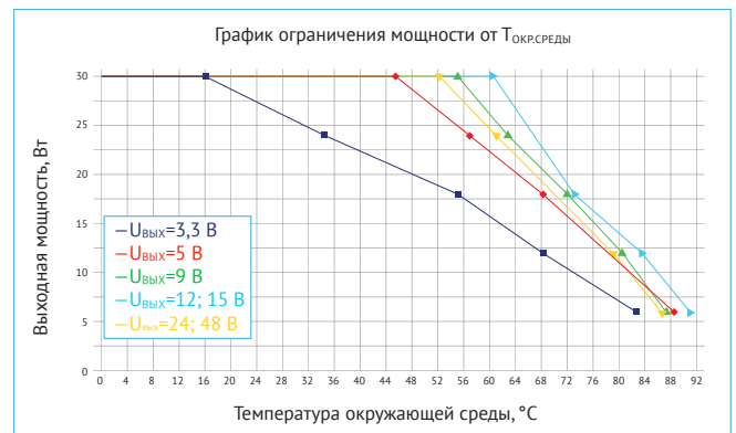
Рис. 26. График ограничения мощности от T_{окр.среды} без применения внешнего радиатора. Для модулей VDRI30W с входной сетью «W», при U_{BX}=48 В .
