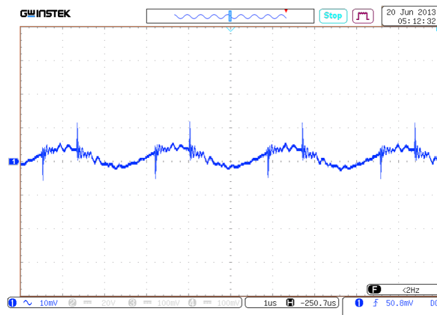
Рис. 34. Пульсации U_{ВЫХ.НОМ} .
