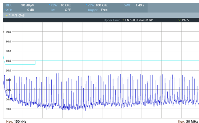
Рис. 46. Спектрограмма работы VDRI30B24 по схеме включения [Рис. 4], измерения произведены в соответствии с EN 55032 Class B (0,15–30 МГц).
