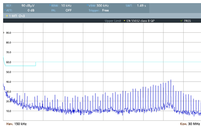
Рис. 44. Спектрограмма работы VDRI30B05 по схеме включения [Рис. 4], измерения произведены в соответствии с EN 55032 Class B (0,15–30 МГц).
