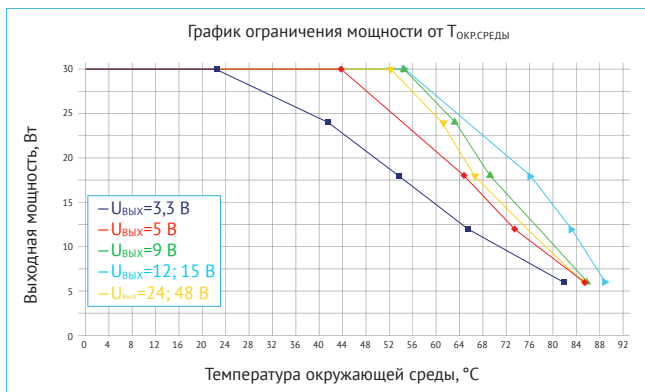
Рис. 25. График ограничения мощности от T_{окр.среды} без применения внешнего радиатора. Для модулей VDRI30B с входной сетью «В», при U_{BX}=24 В .
