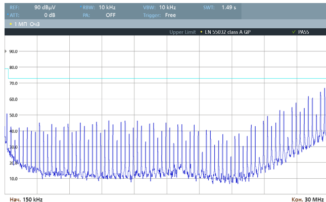
Рис. 49. Спектрограмма работы VDRI30W48 по схеме включения [Рис. 3], измерения произведены в соответствии с EN 55032 Class A (0,15–30 МГц).
