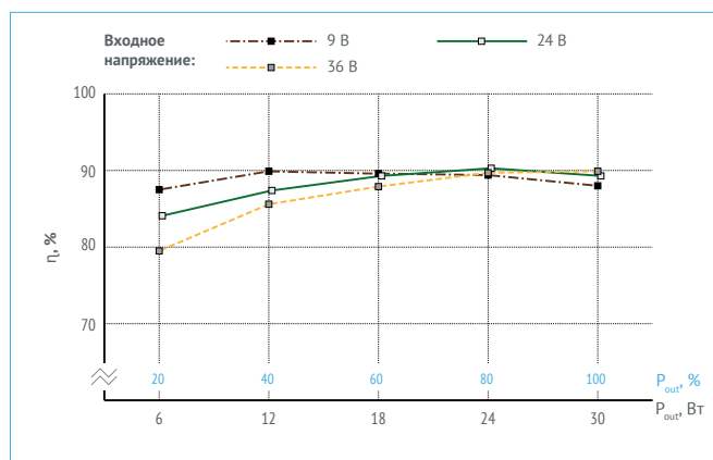
Рис. 15. КПД для VDRI30B15.
