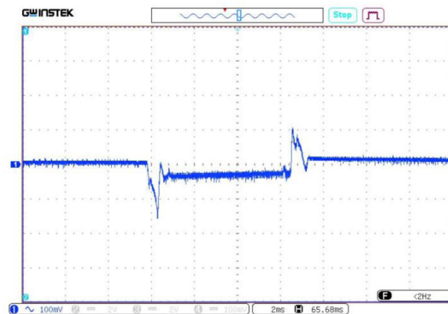
Рис. 28. Осциллограмма переходного отклонения выходного напряжения при скачкообразном изменении выходного тока с 50% до 100% и со 100% до 50%.
