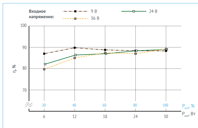
Рис. 16. КПД для VDRI30B24.
