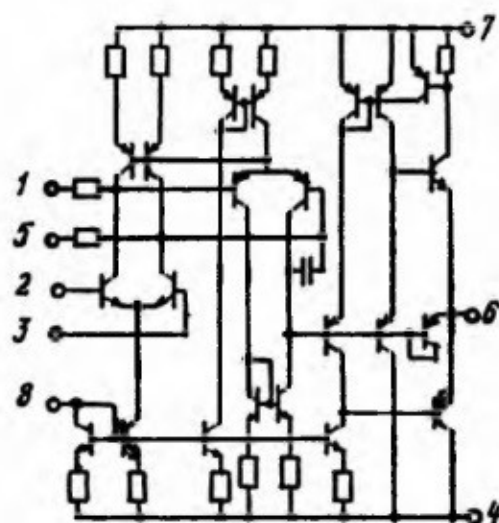
Принципиальная схема ИМС КР1407УД2
