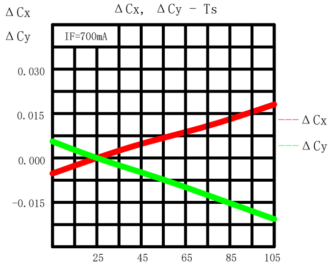
温度-色坐标漂移曲线
