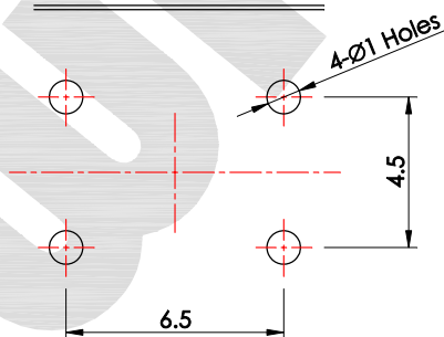
P.C.B. LAND PATTERN
