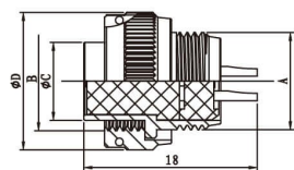
不带尾附电缆插头 Cable plug without tail
